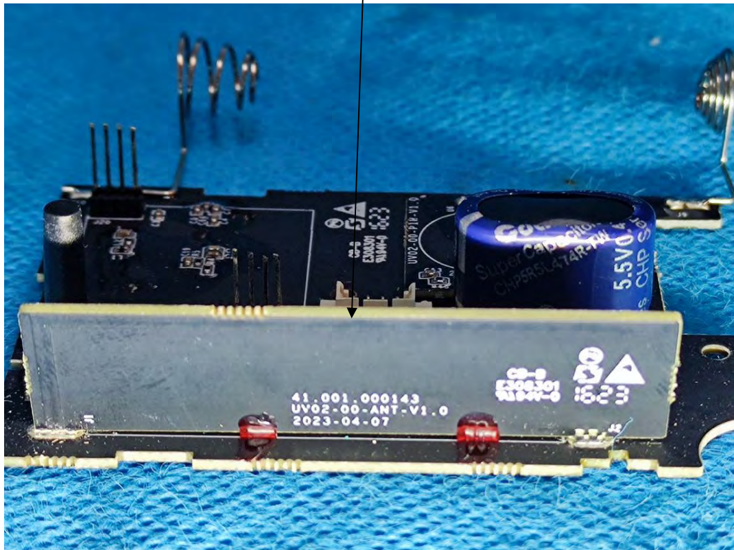
Lora ANT
