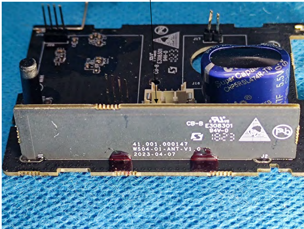
Lora Antenna
