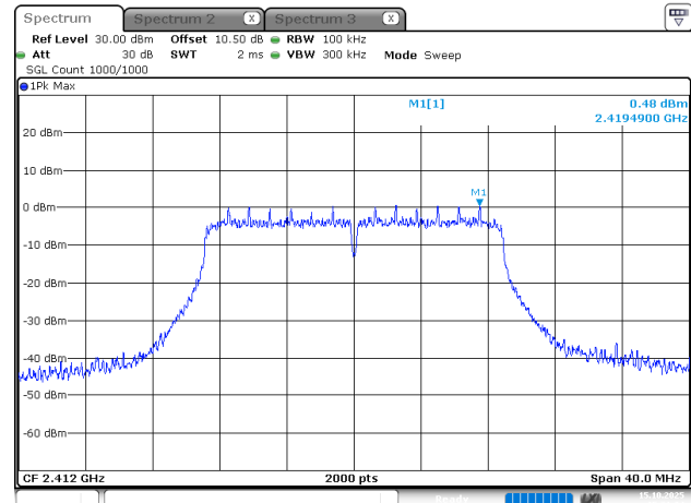
802.11n20_2412MHz
