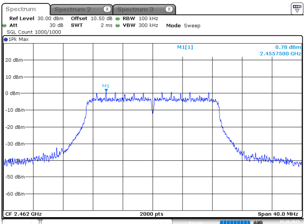
802.11n20_2462MHz
