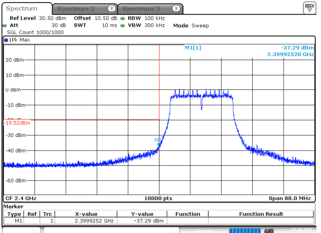
802.11n20_2412MHz
