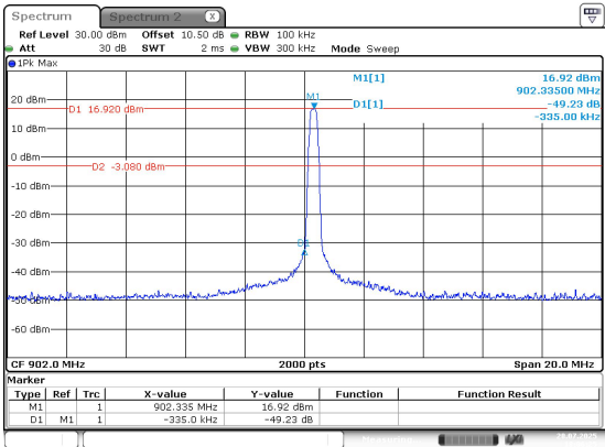
Left_Single
