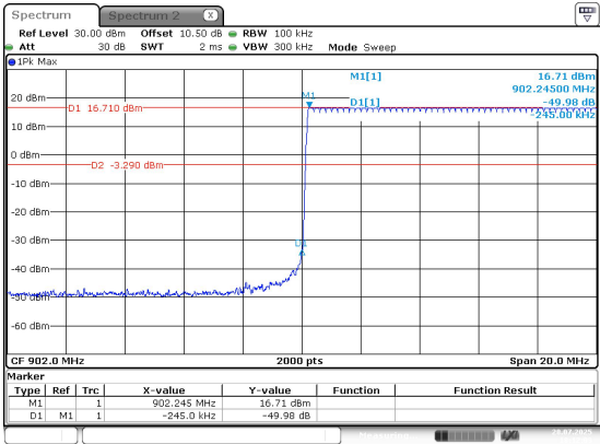
Left_Hopping
