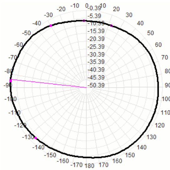
915.0MHz Total(E1),
