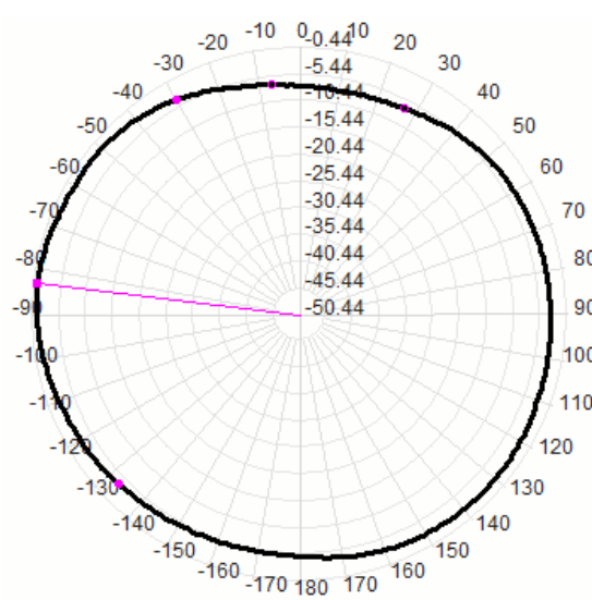
902.0MHz Total(E1)
