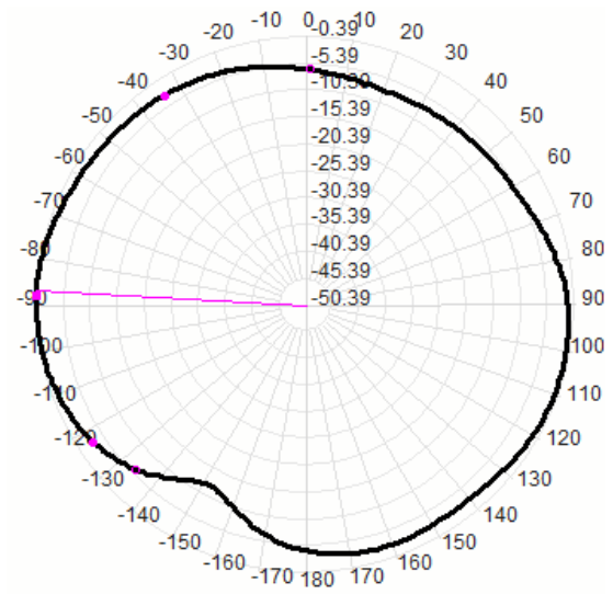
915.0MHz Total(E2),
