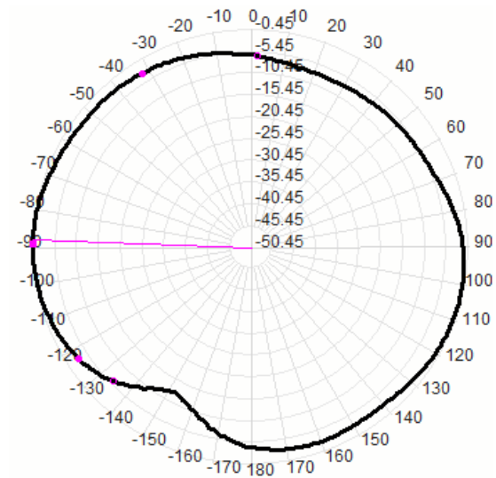
928.0MHz Total(E2)
