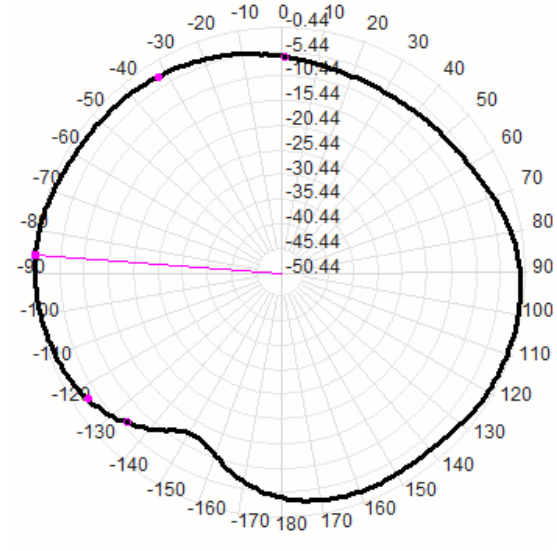
902.0MHz Total(E2)
