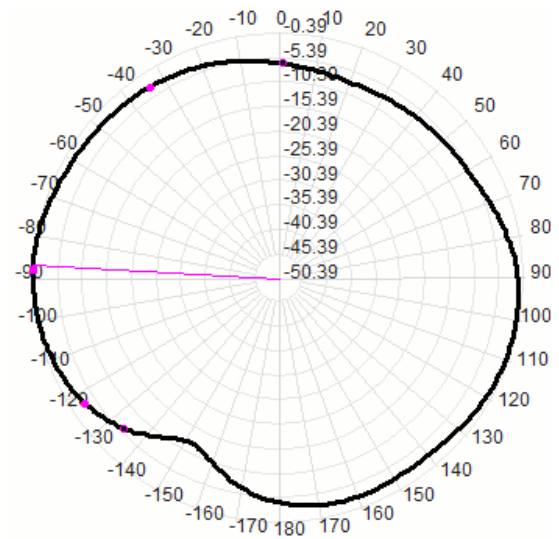
915.0MHz Total(E2),
