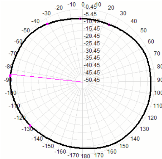
928.0MHz Total(E1)
