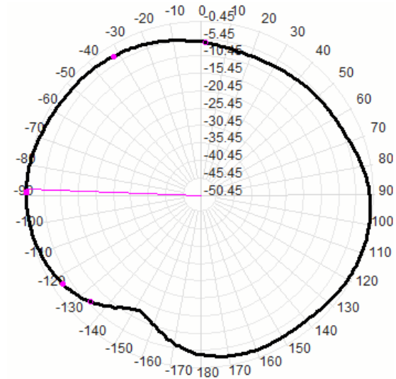
928.0MHz Total(E2)
