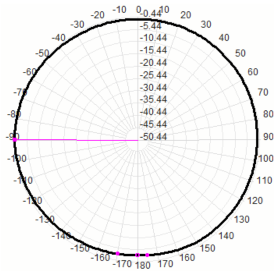
902.0MHz Total(H)
