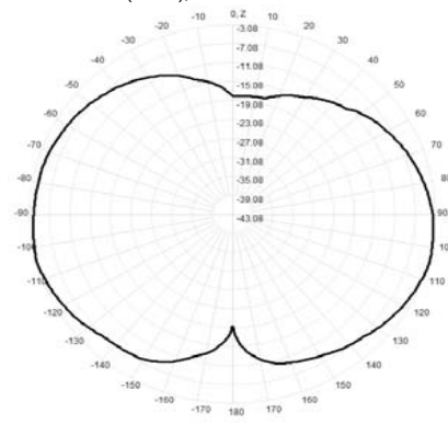
921.0MHz Total(E2-YZ), Max= -3.24dBi
