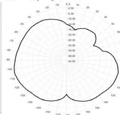
908.0MHz Total(E1-XZ), Max= -4.41dBi
