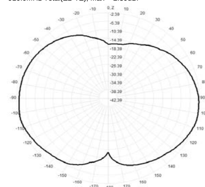
910.0MHz Total(E2-YZ), Max= -2.39dBi
