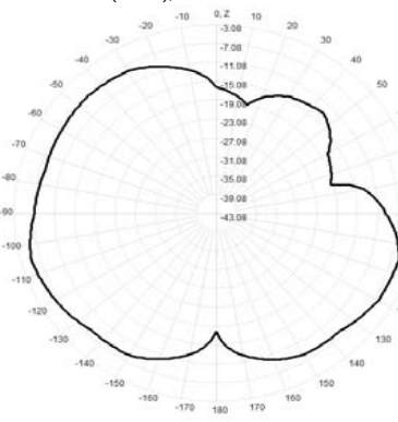
921.0MHz Total(E1-XZ), Max= -5.30dBi
