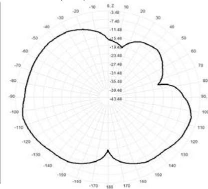
925.0MHz Total(E1-XZ), Max= -5.57dBi
