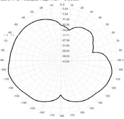
922.0MHz Total(E1-XZ), Max= -5.36dBi
