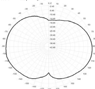
905.0MHz Total(E2-YZ), Max= -2.46dBi
