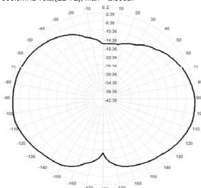
906.0MHz Total(E2-YZ), Max= -2.36dBi
