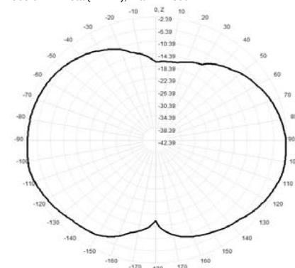
908.0MHz Total(E2-YZ), Max= -2.39dBi
