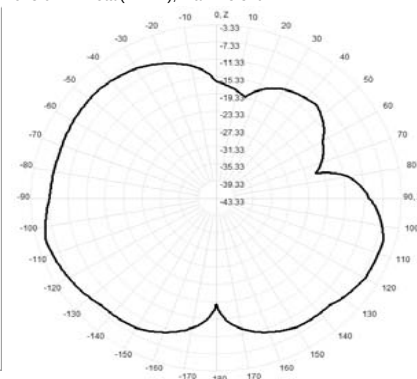
923.0MHz Total(E1-XZ), Max= -5.34dBi
