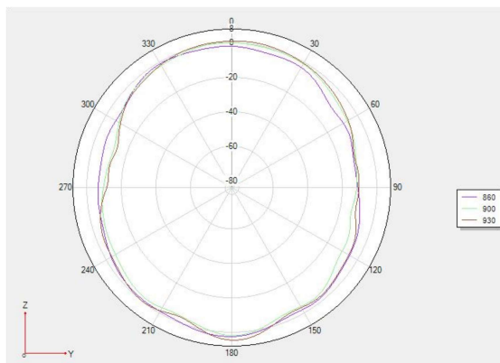
Phi 90 2D图
