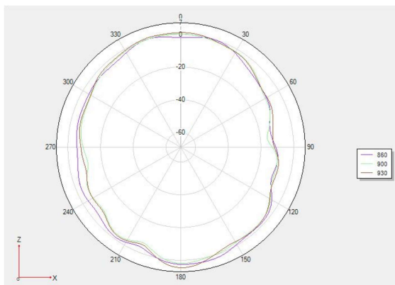
Phi 0 2D图
