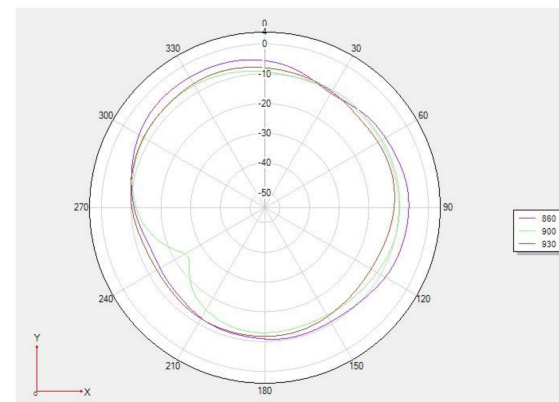
Theta 90 2D图
