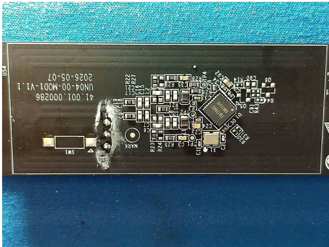
NFC Antenna(only RX)
