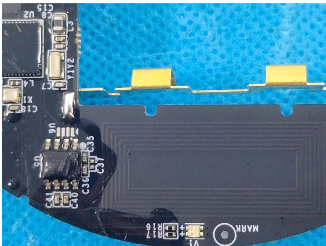
LoRa Antenna
