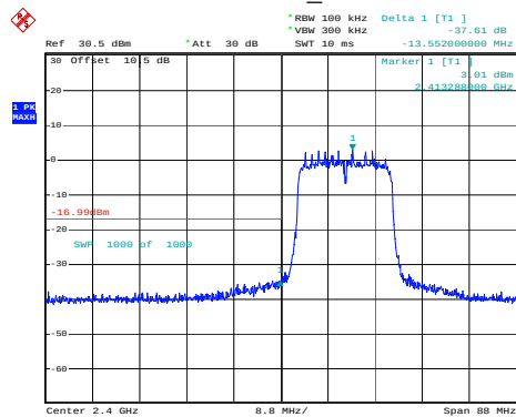
802.11n20_2412MHz
