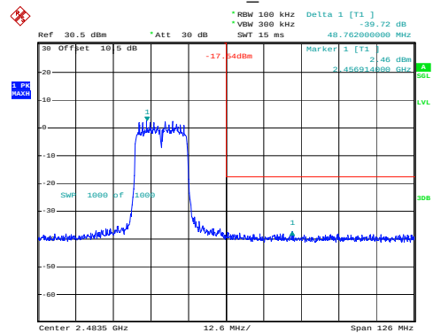
802.11n20_2462MHz
