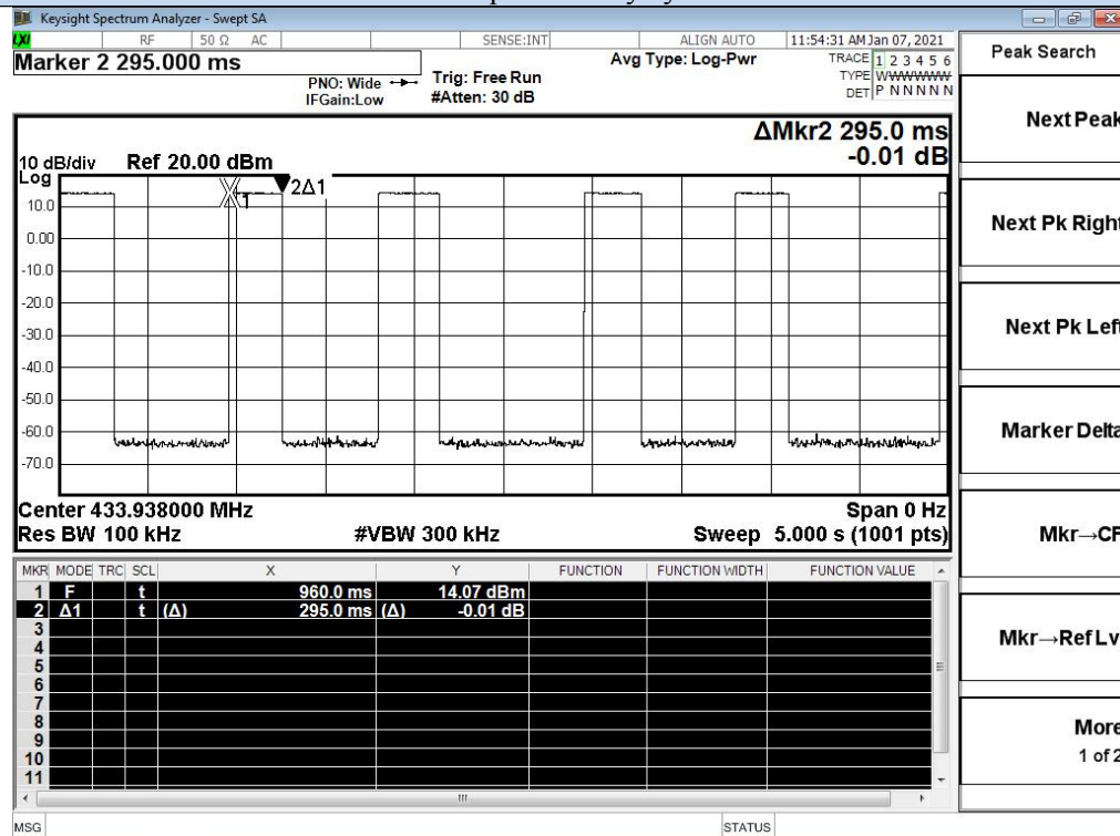
Fig.1(Pulse Period exceed 100ms)
