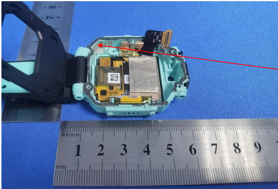
GSM/WCDMA/LTE antenna
