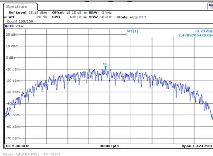
BLE_BT4.0_Ant1_2480
