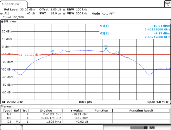
RF4CE_Ant1_2402 MHz
