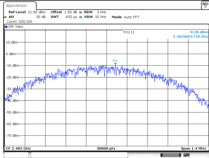
RF4CE_Ant1_2402 MHz
