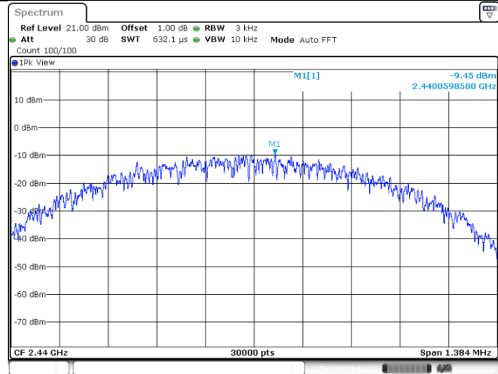
RF4CE_Ant1_2440 MHz
