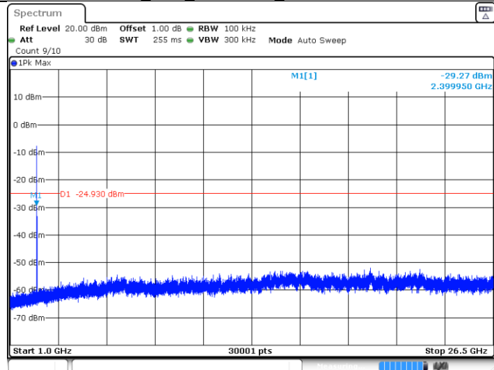
RF4CE_Ant1_2402 MHz_1000~26500 MHz
