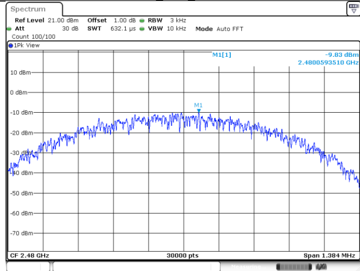
RF4CE_Ant1_2480 MHz
