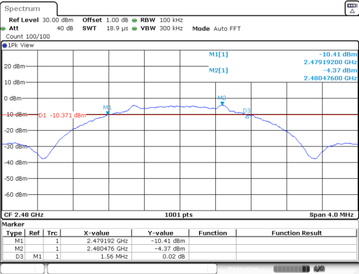
RF4CE_Ant1_2480 MHz
