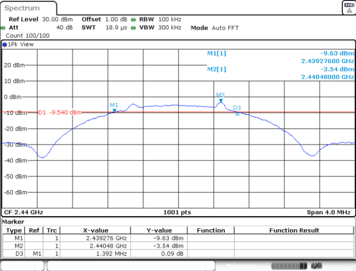
RF4CE_Ant1_2440 MHz
