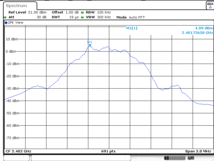
BLE BT5.0 Ant1 2402 MHz MHz_0~Reference
