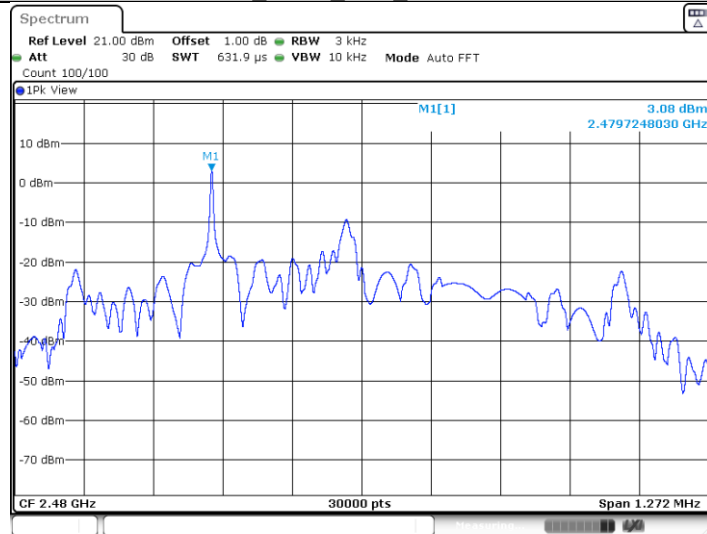
BLE_BT5.0_Ant1_2480 MHz
