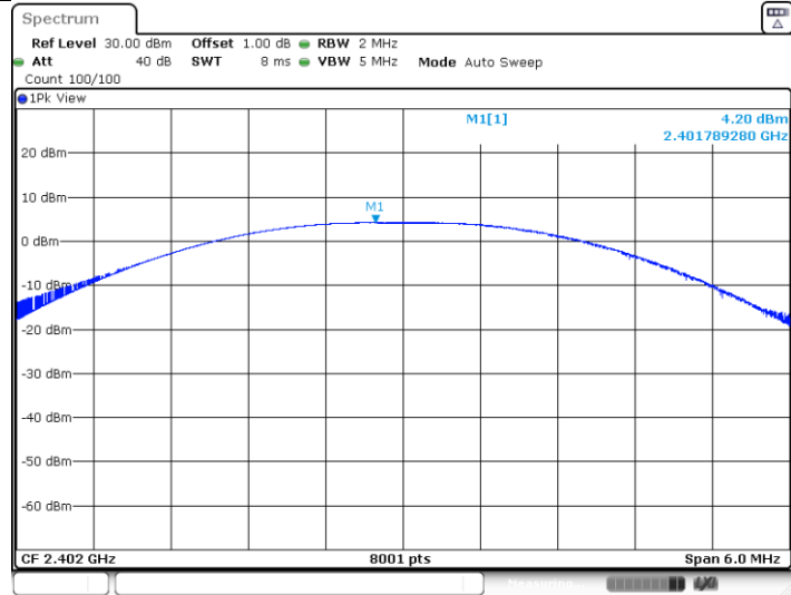
BLE_BT5.0_Ant1_2402 MHz
