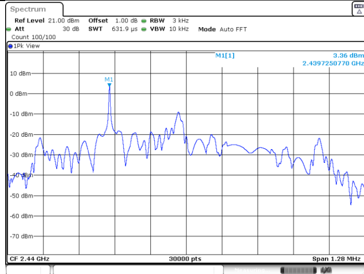
BLE_BT5.0_Ant1_2440 MHz
