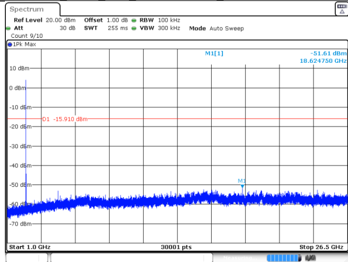
BLE BT5.0 Ant1 2402 MHz MHz_1000~26500 MHz
