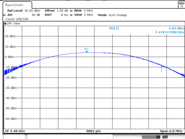
BLE_BT5.0_Ant1_2480 MHz
