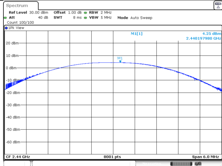
BLE_BT5.0_Ant1_2440 MHz
