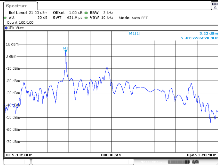
BLE_BT5.0_Ant1_2402 MHz
