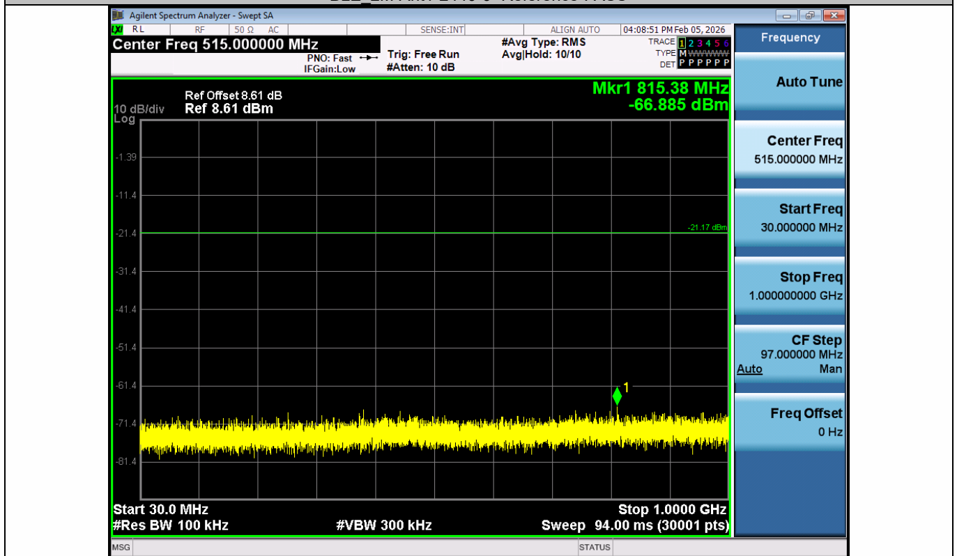
BLE 2M-Ant1-2440-30~1000-PASS
