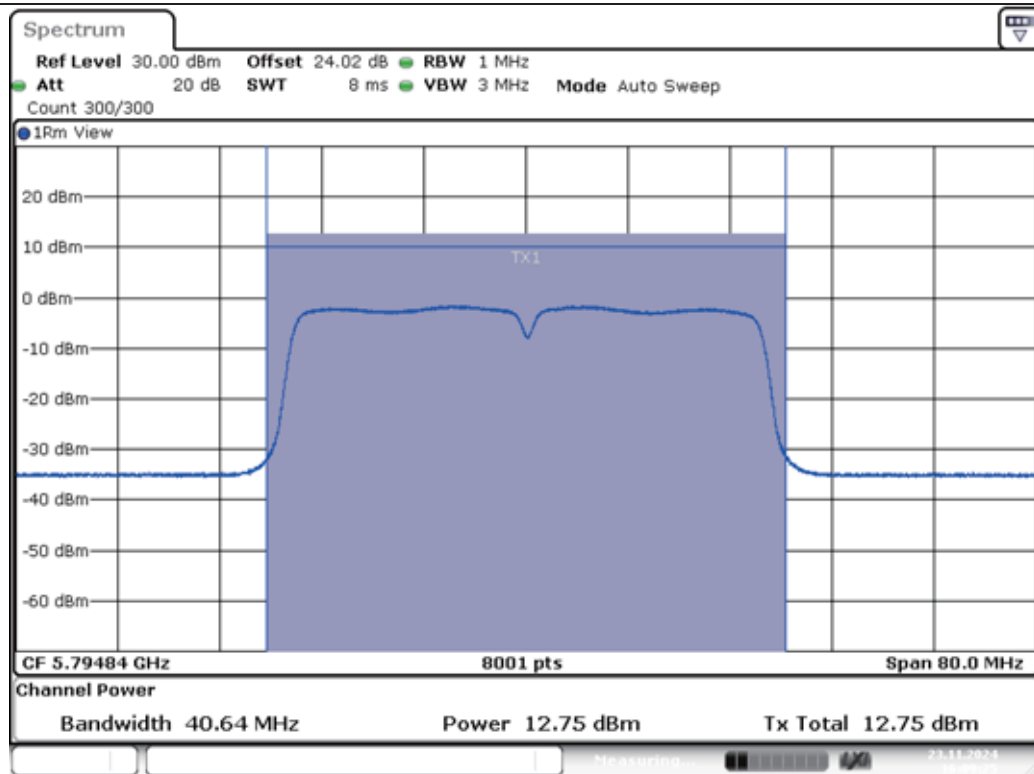
11N40MIMO-Ant1-5795-PASS
