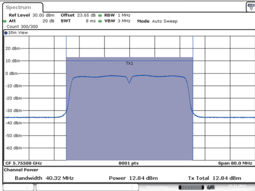
11N40MIMO-Ant1-5755-PASS
