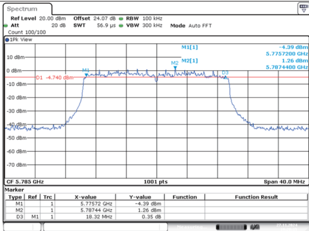
11AX20MIMO-Ant1-5785-PASS
