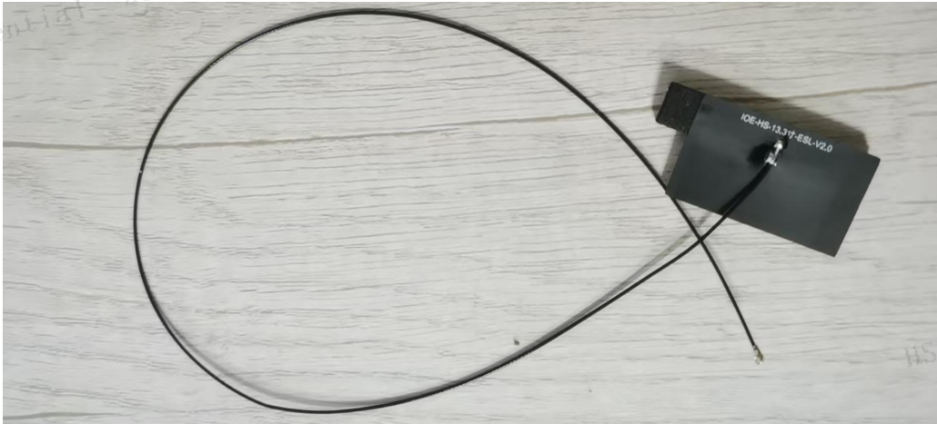
HS-13.3 寸-ESL 天线 FPC 黑色 TO IPEX 三代 Cable OD0.81mm 黑色 L370mm
