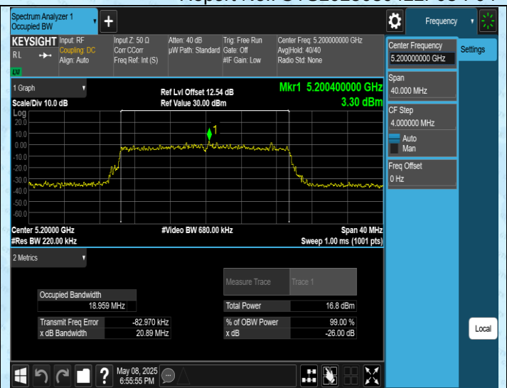
11AX20SISO-Ant1-5200
