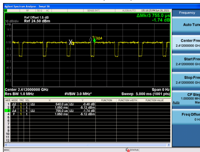
802.11n(20MHz)
