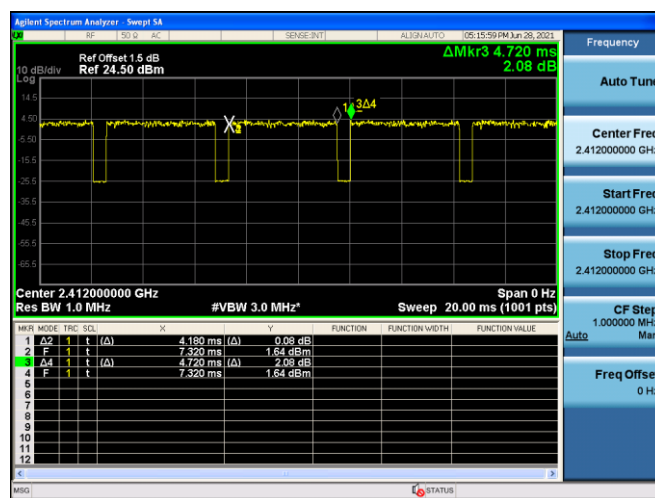
802.11n(20MHz)
