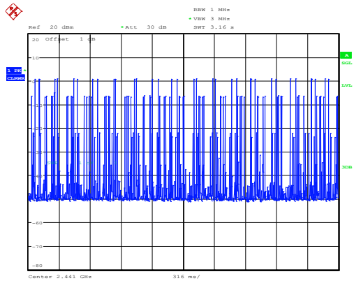
DH1_Hopping
