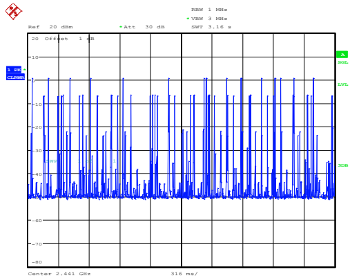
DH3_Hopping
