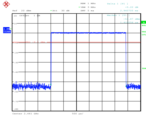
DH5_Hopping
