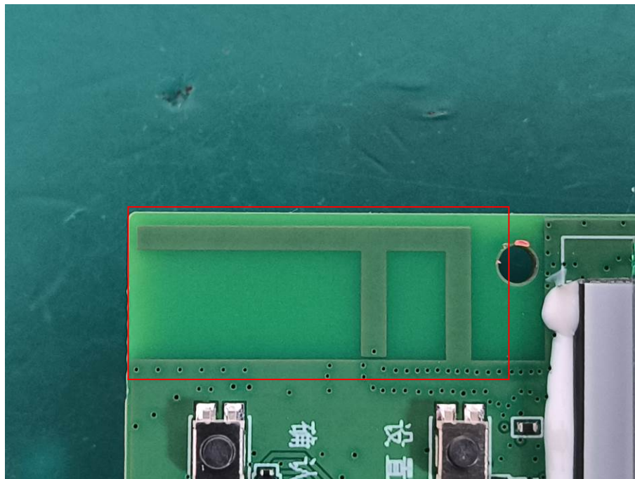
BLE/Wi-Fi ANT
