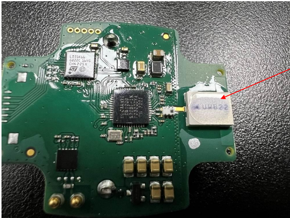
UWB antenna
