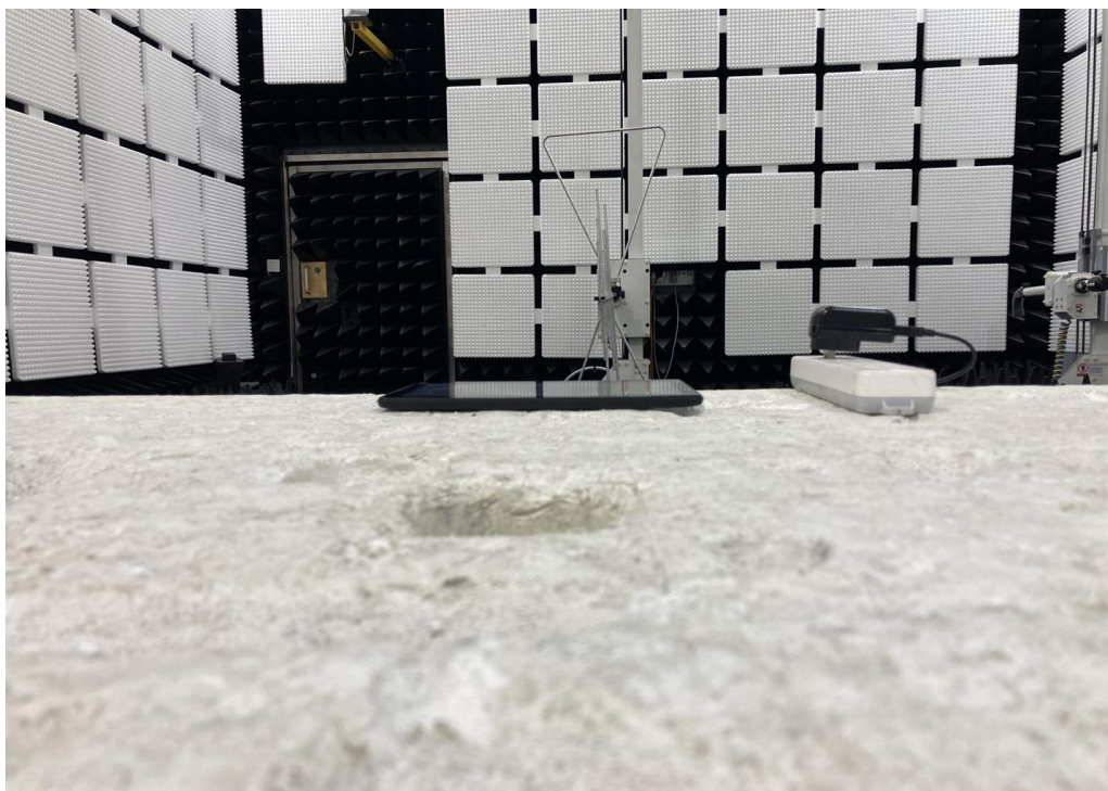
Fig. 1 (Below 1GHz)
