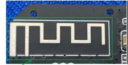
BLE ANT
