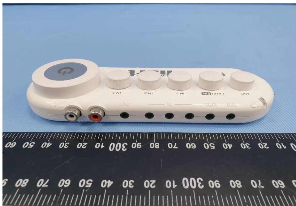
EUT Photo (6)
