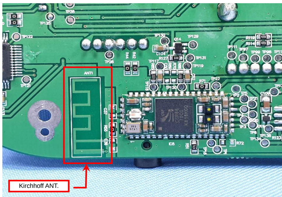
EUT Photo (16)
