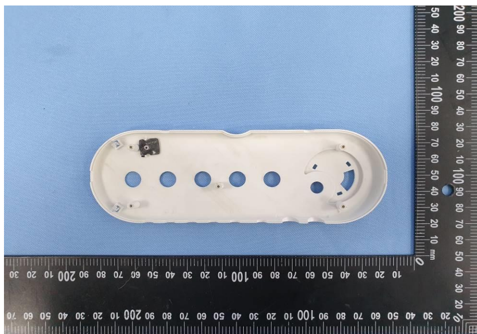
EUT Photo (8)
