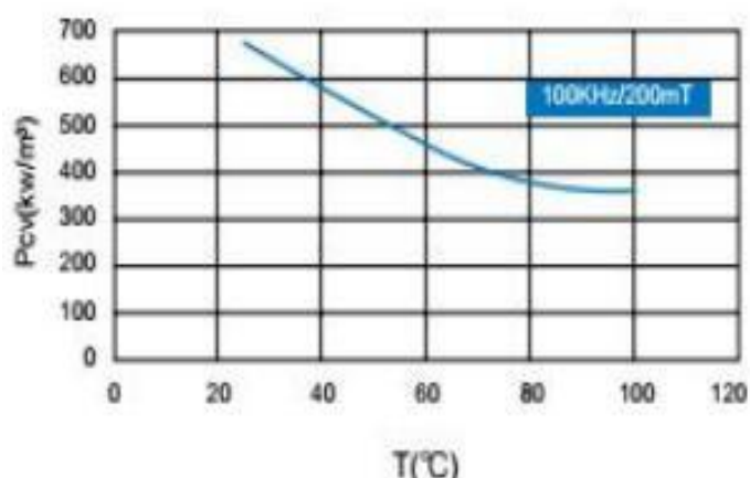
Pcv—T 曲线
