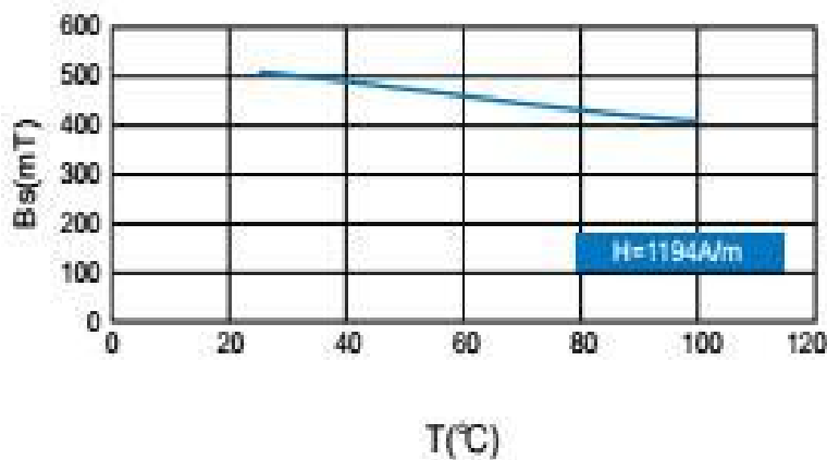
Bs—T 曲线
