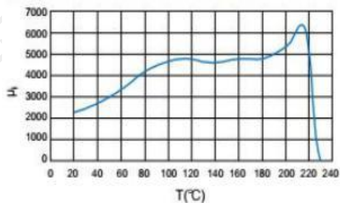
μi—T 曲线
