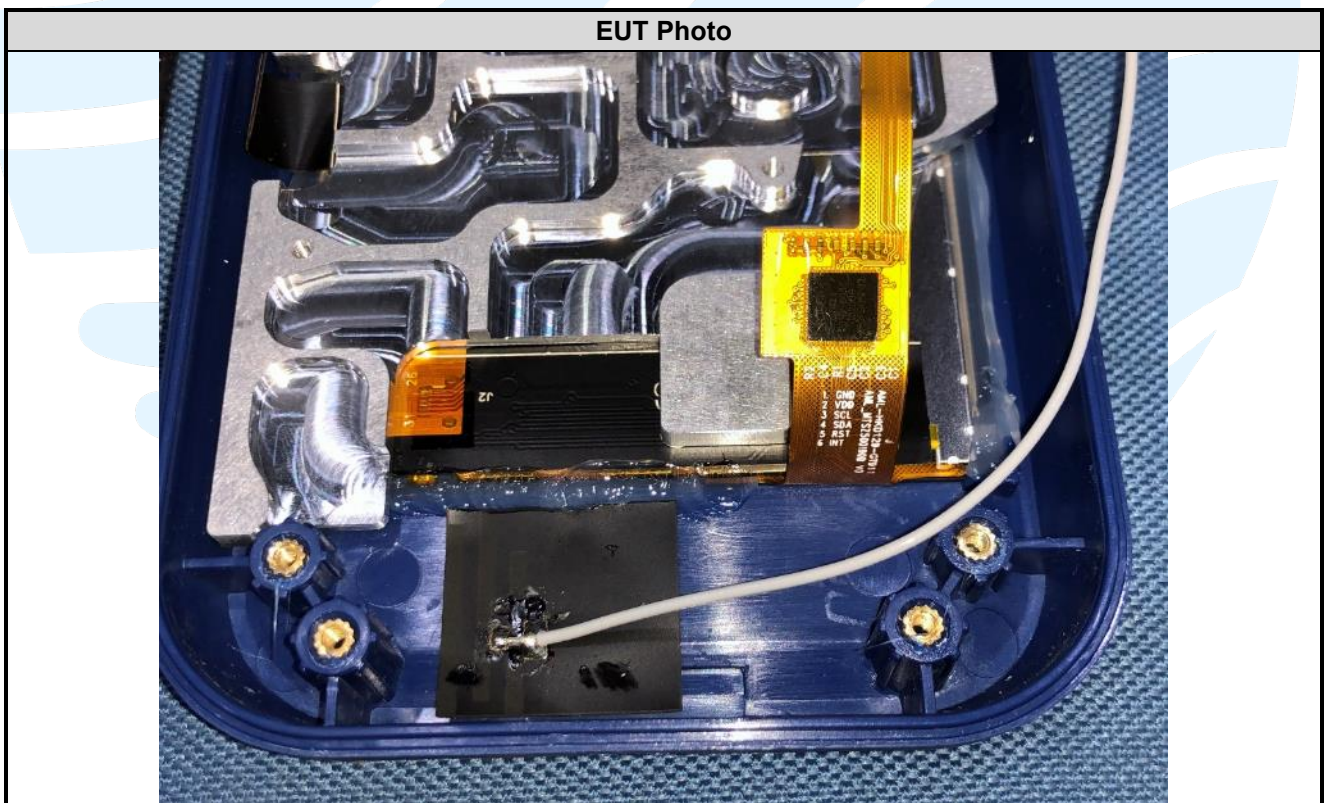
Wi-Fi/BT Antenna
