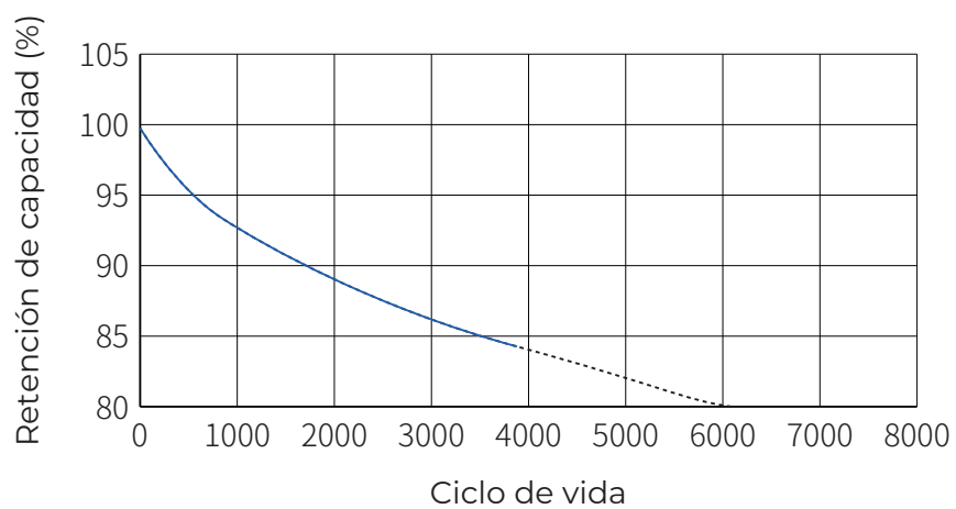
Ciclos de vida a 0,5C, 77 °F (25 °C)
