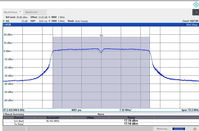
11N40ISO-Ant1-2422-PASS
