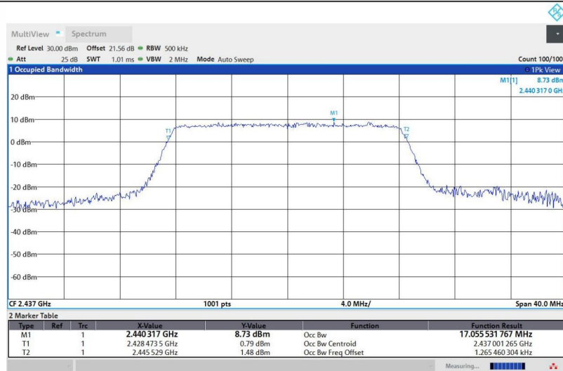
11G-Ant1-2437
