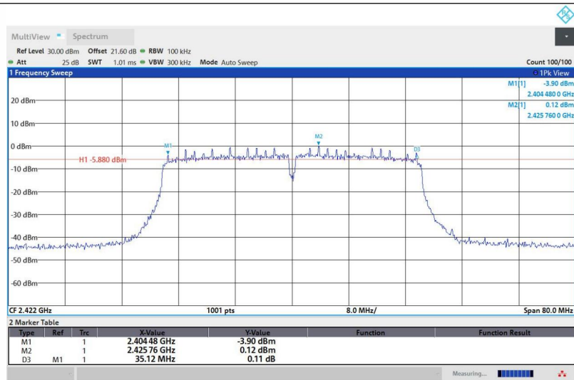
11N40ISO-Ant1-2422-PASS
