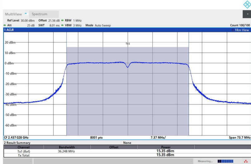
11N40ISO-Ant1-2437-PASS
