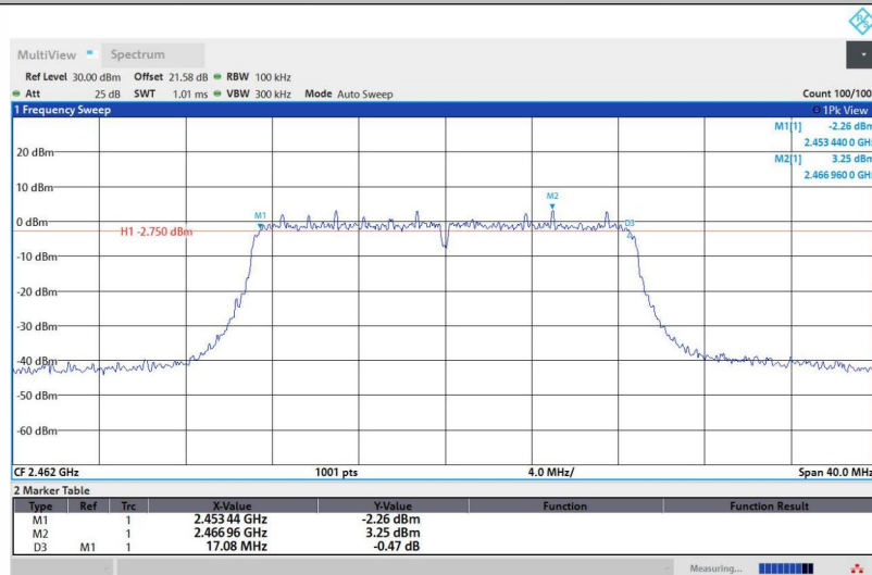
11N20ISO-Ant1-2462-PASS
