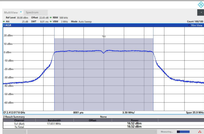
11N20ISO-Ant1-2412-PASS
