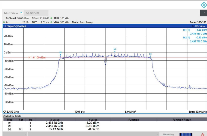
11N40ISO-Ant1-2452-PASS
