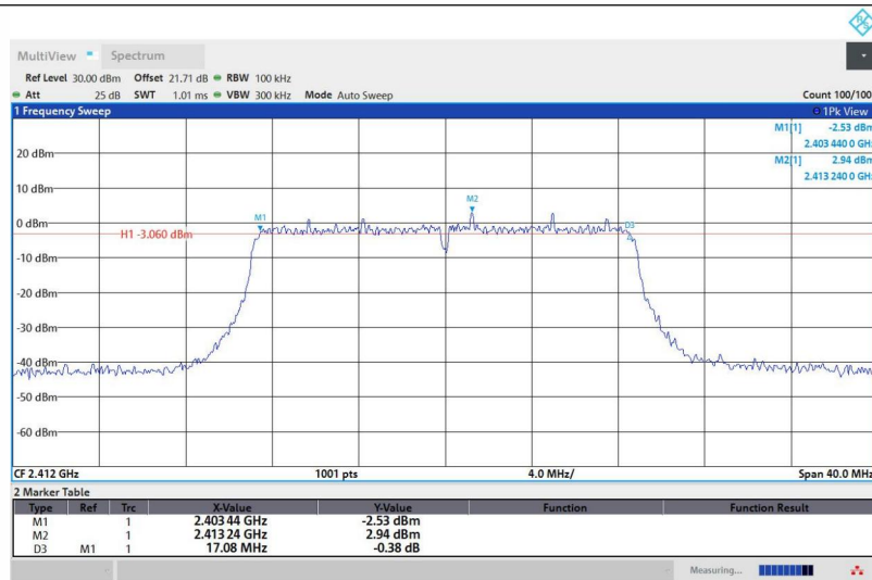
11N20ISO-Ant1-2412-PASS
