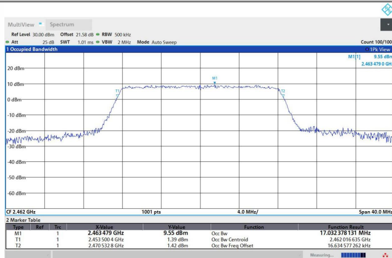
11G-Ant1-2462
