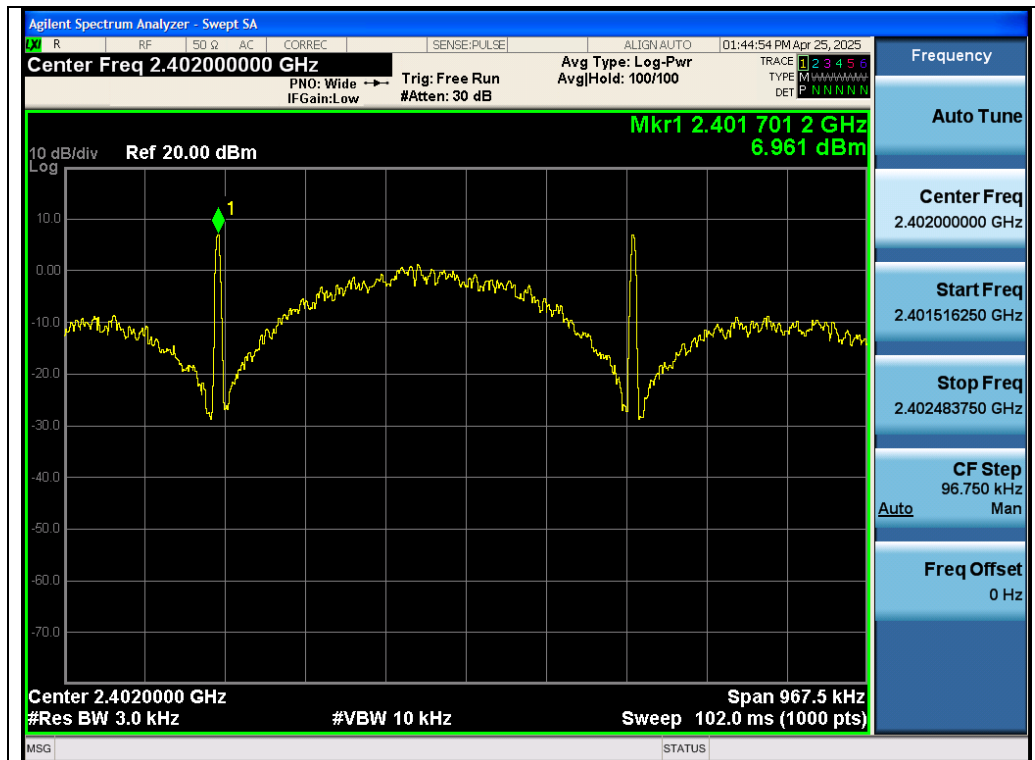
Test_Graph_LE500K_ANT1_2402_500Kbps_PSD
