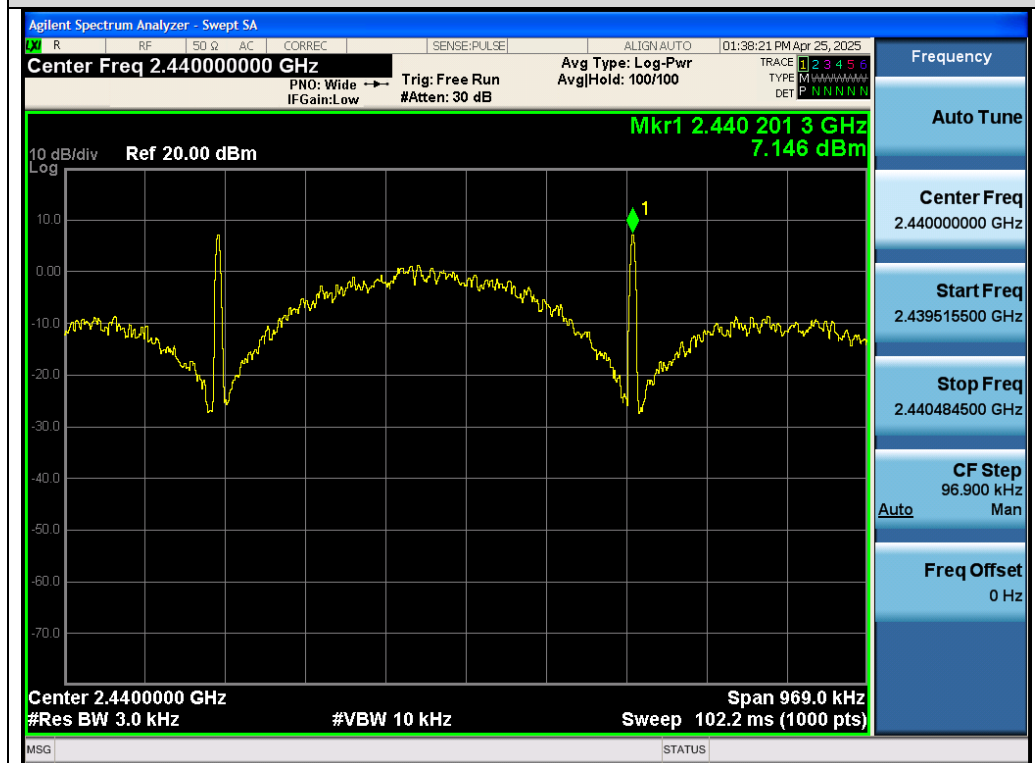
Test_Graph_LE500K_ANT1_2440_500Kbps_PSD
