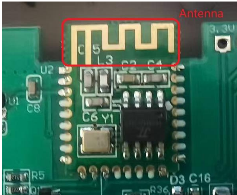
BLE module view
