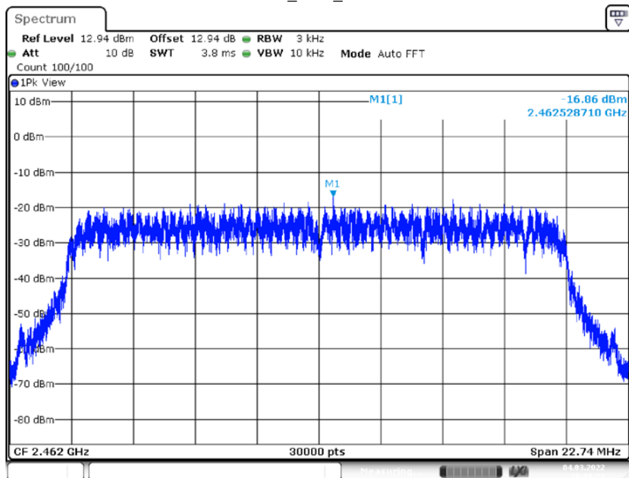
11G_Ant1_2462
