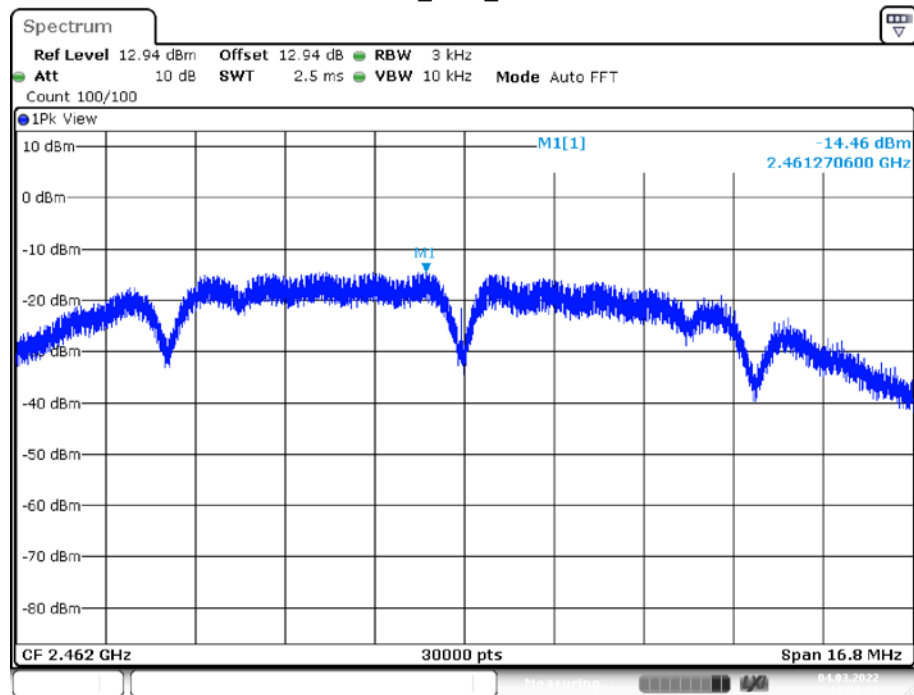
11B_Ant1_2462
