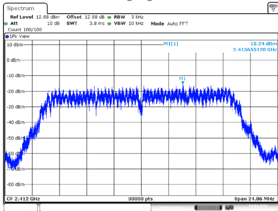
11G_Ant1_2412
