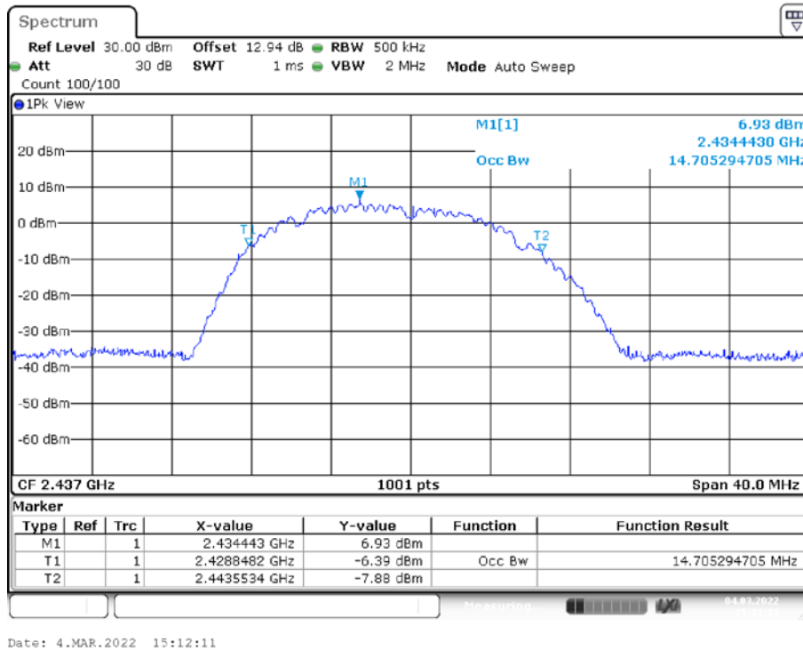
11B_Ant1_2437
