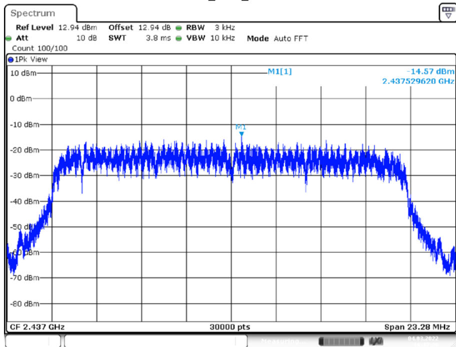
11G_Ant1_2437
