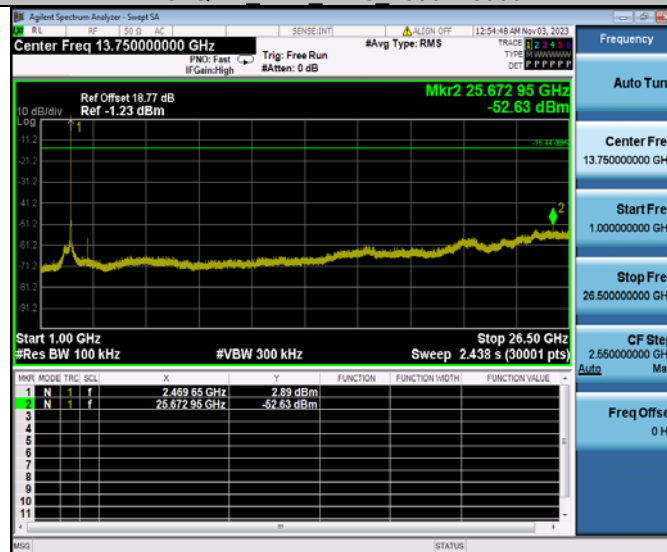
64QAM Ant2 2470 1000~26500
