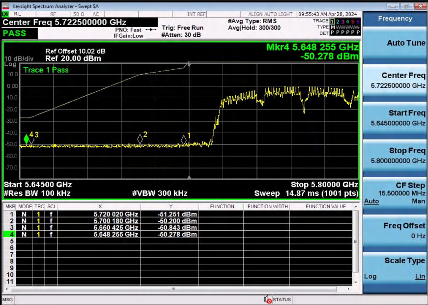
11AC80SISO-5775-PASS
