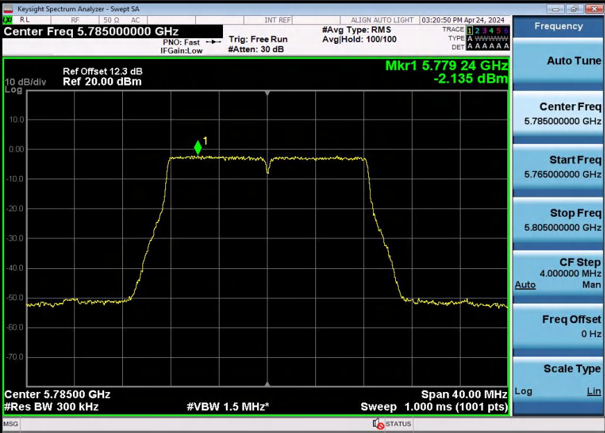
11N20SISO-5785-PASS
