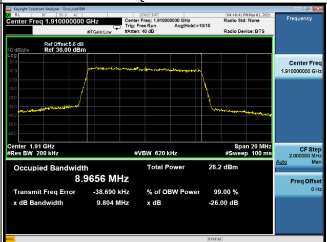
16QAM-26640
