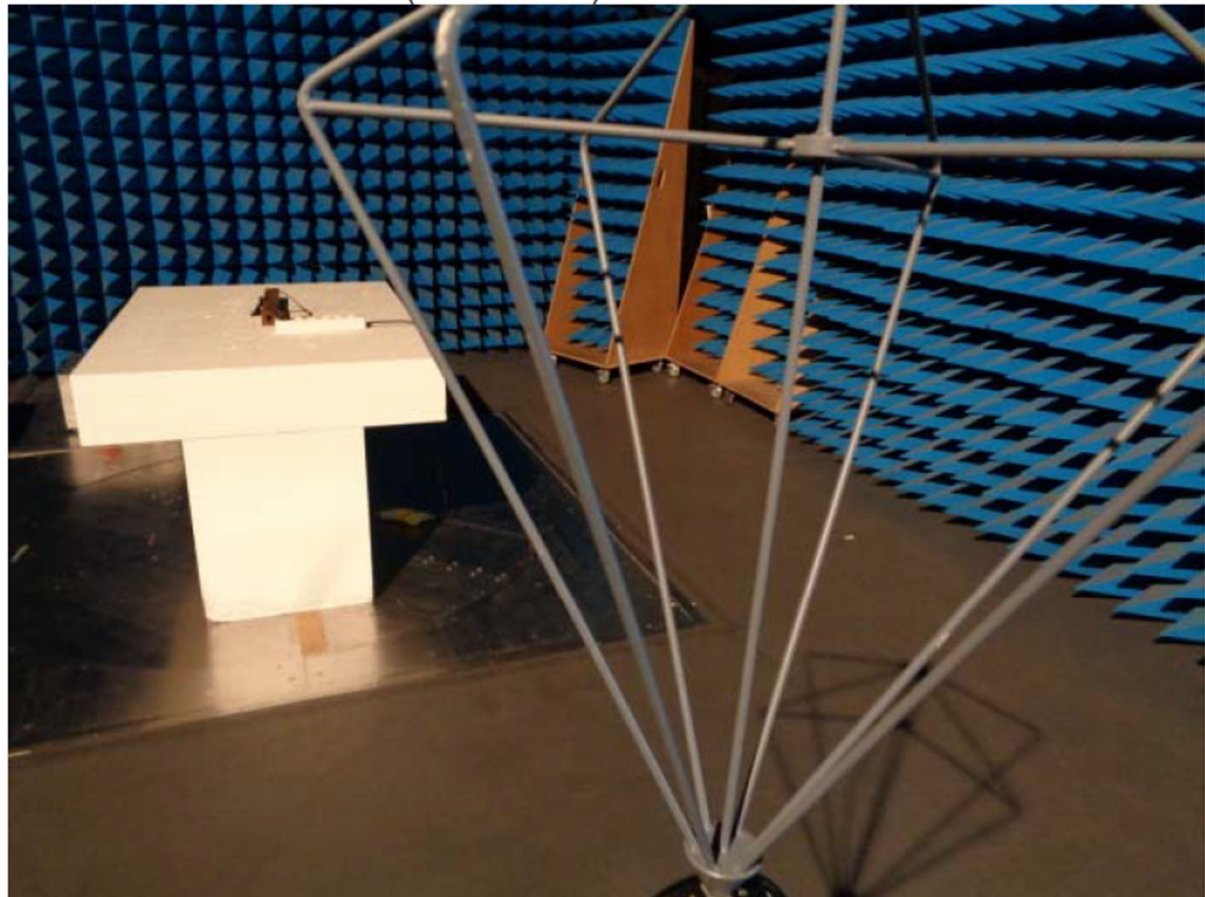
Photo : radiates emission (30-200MHz)
