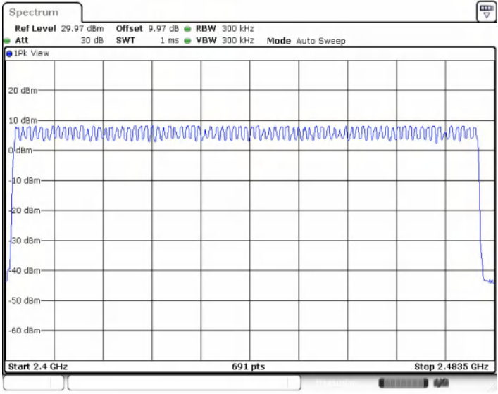
2DH5_Ant1_Hop
