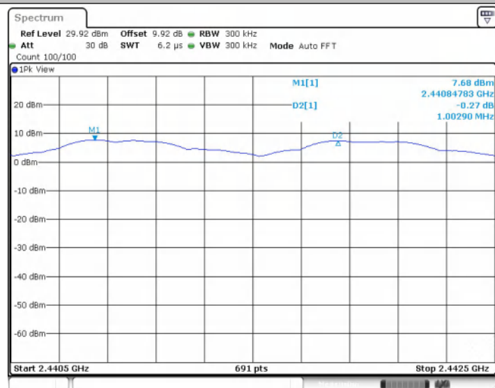
2DH5_Ant1_Hop
