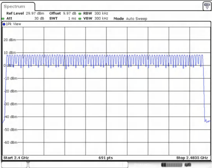
DH5_Ant1_Hop
