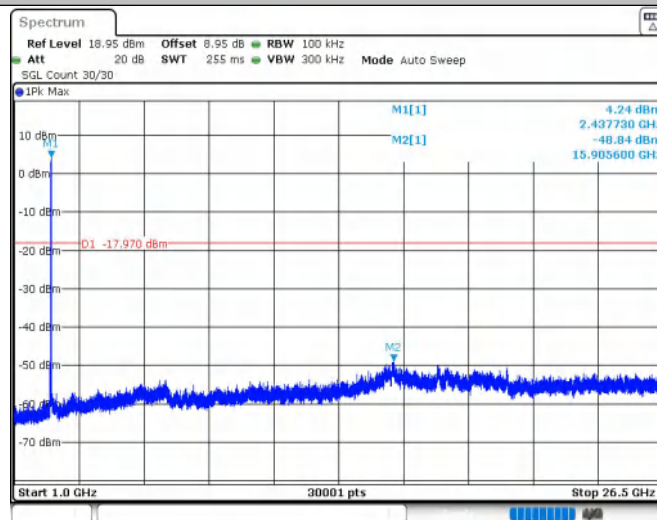
11B_Ant1_2437_1000~26500
