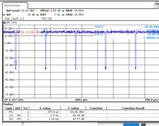
11N20MIMO_Ant1_2437
