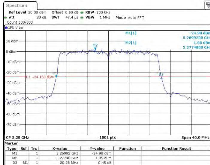
11AX20MIMO_Ant0_5280
