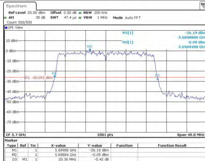
11N20MIMO_Ant0_5700
