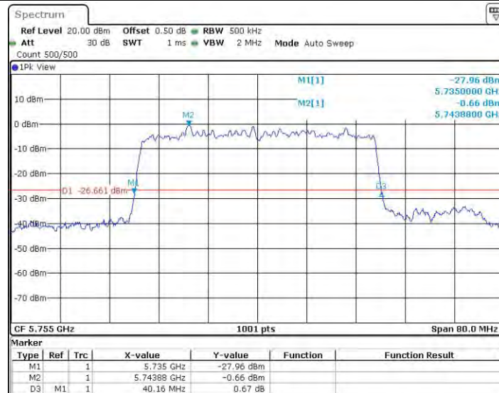
11AX40MIMO_Ant1_5755
