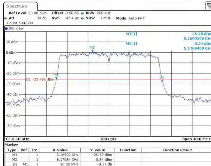
11AX20MIMO_Ant0_5180
