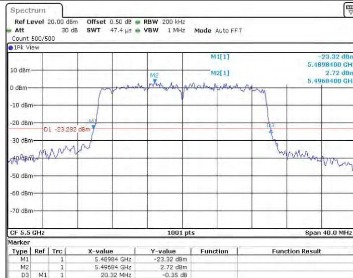
11N20MIMO_Ant1_5500
