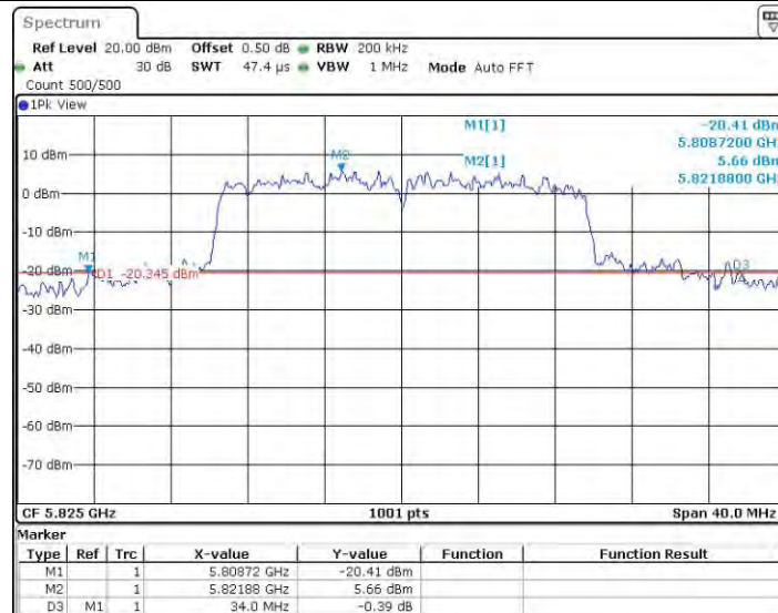
11N20MIMO_Ant0_5825
