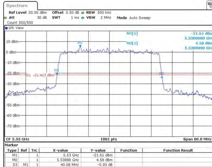
11AX40MIMO_Ant1_5550
