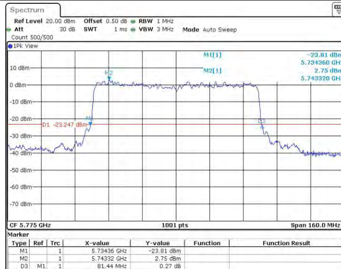
11AX80MIMO_Ant0_5775
