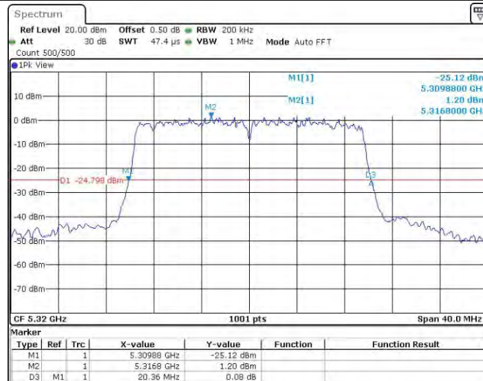
11N20MIMO_Ant0_5320
