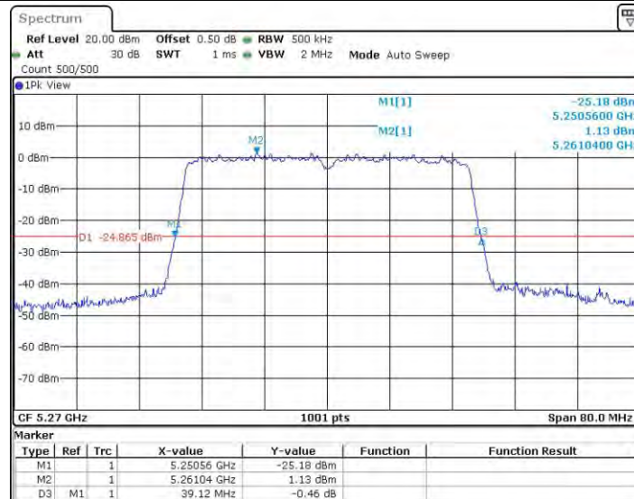
11N40MIMO_Ant0_5270
