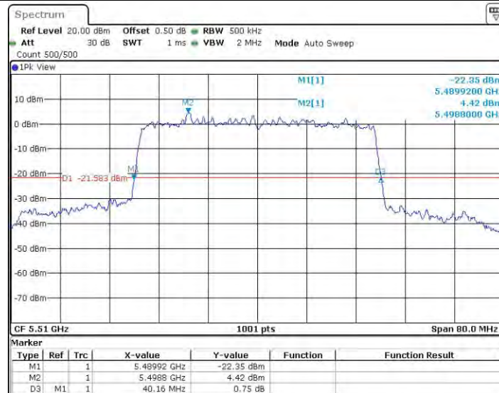
11AX40MIMO_Ant1_5510
