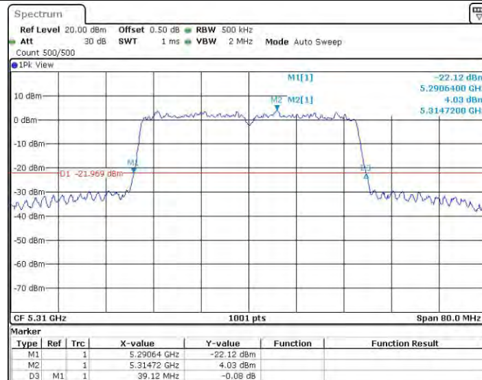
11AC40MIMO_Ant1_5310
