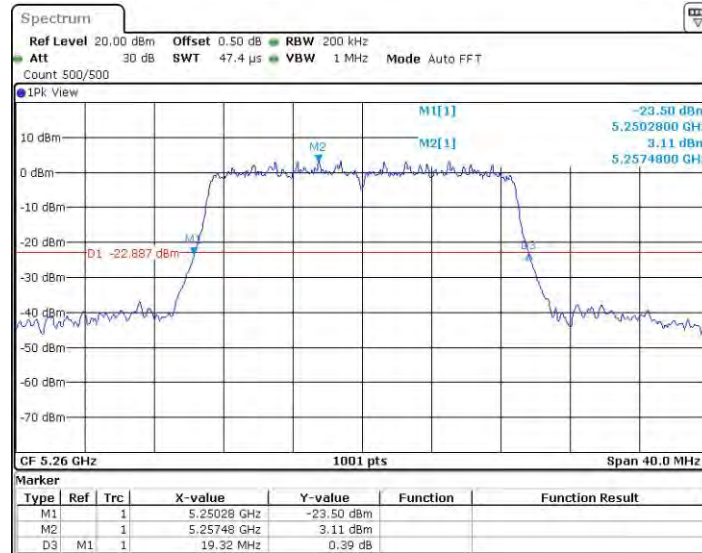
11AC20MIMO_Ant0_5260
