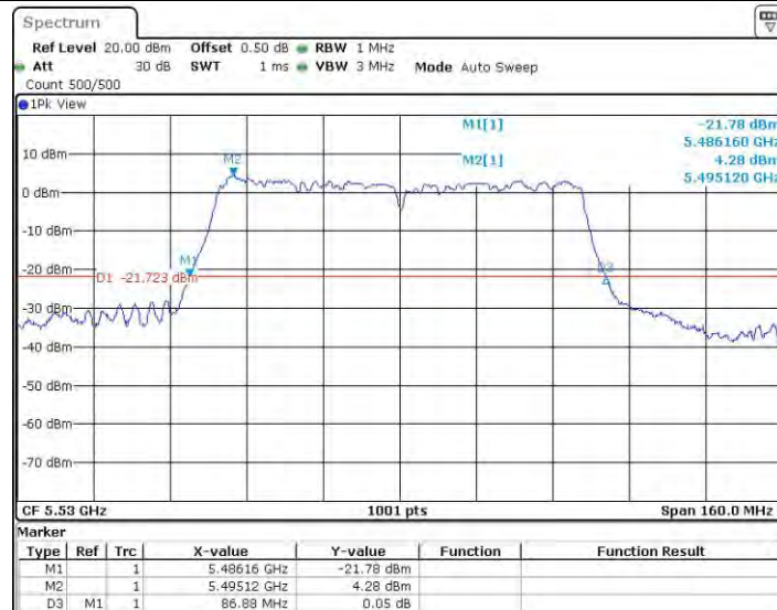
11AC80MIMO_Ant0_5530
