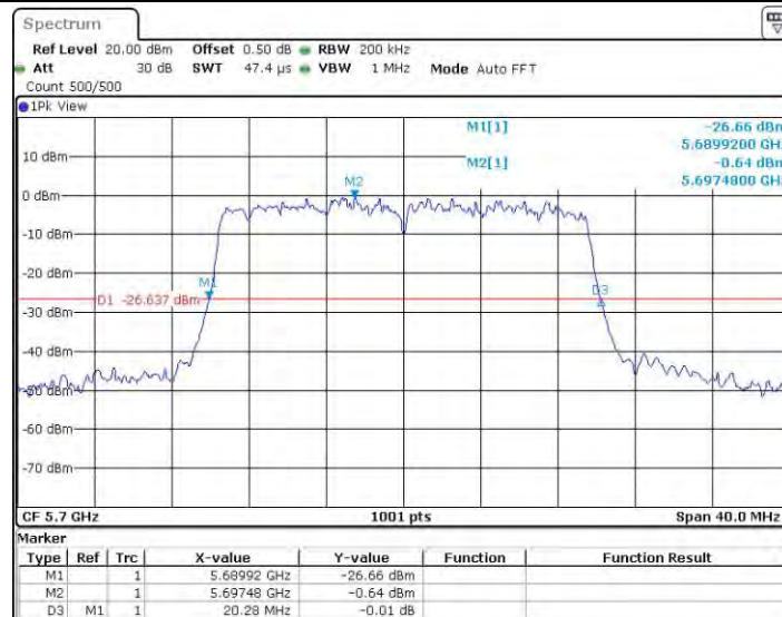
11AX20MIMO_Ant0_5700
