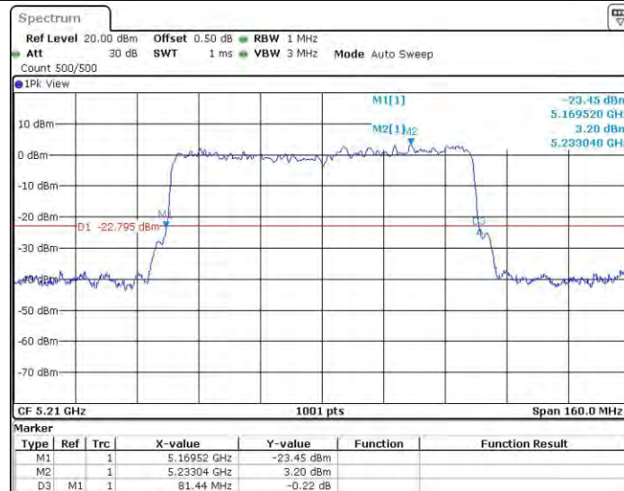
11AX80MIMO_Ant0_5210
