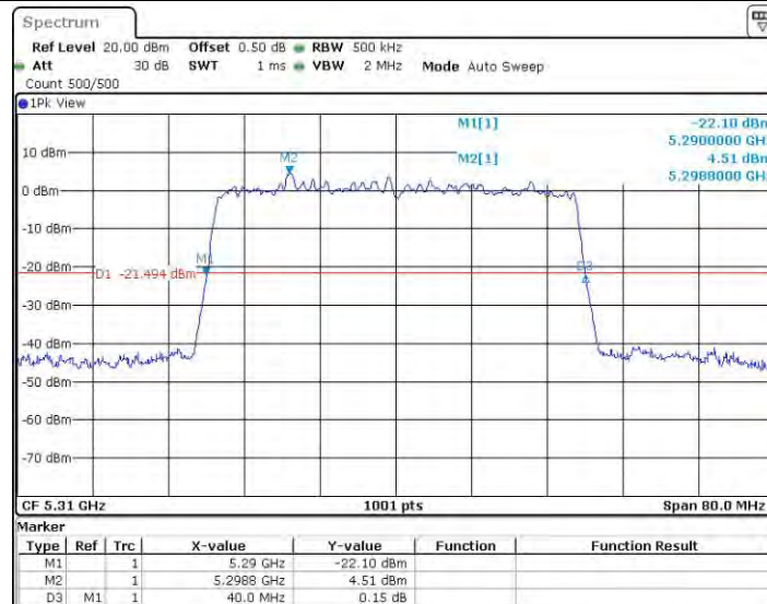
11AX40MIMO_Ant0_5310
