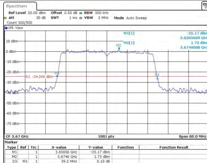
11AC40MIMO_Ant1_5670
