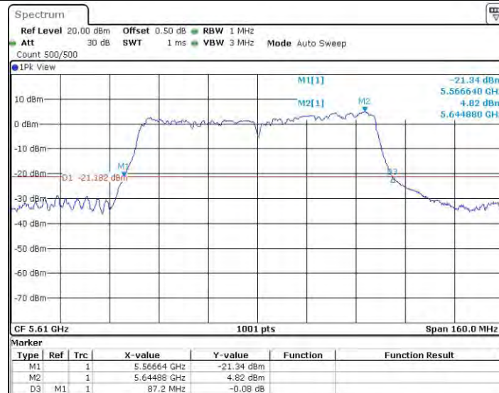
11AC80MIMO_Ant1_5610
