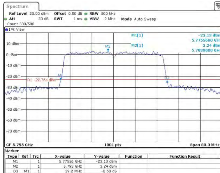
11AC40MIMO_Ant0_5795
