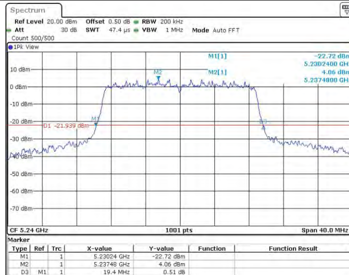
11AC20MIMO_Ant0_5240
