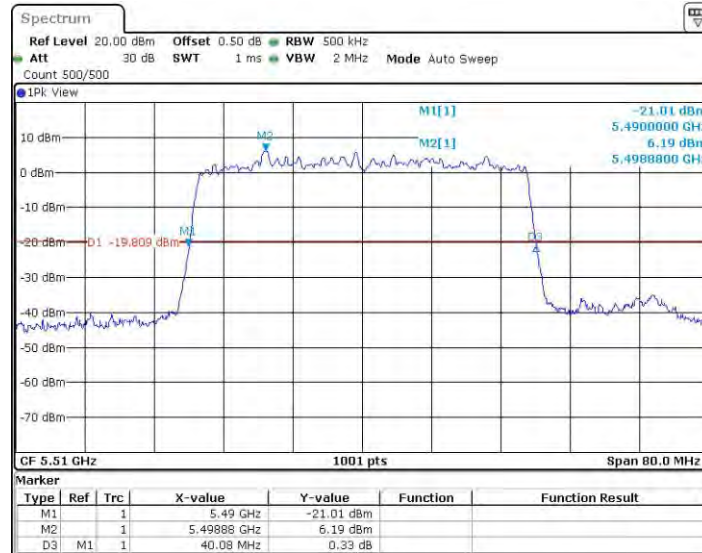
11AX40MIMO_Ant0_5510
