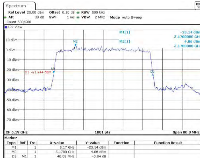
11AX40MIMO_Ant0_5190
