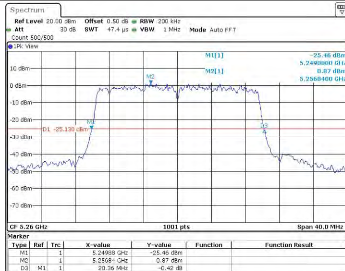
11AX20MIMO_Ant0_5260
