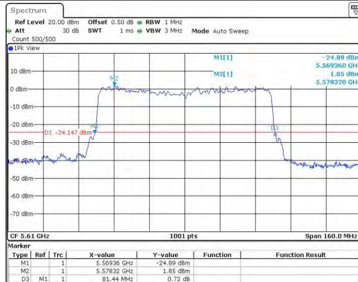
11AX80MIMO_Ant0_5610
