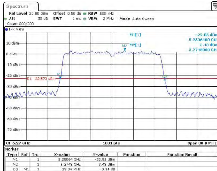
11AC40MIMO_Ant0_5270
