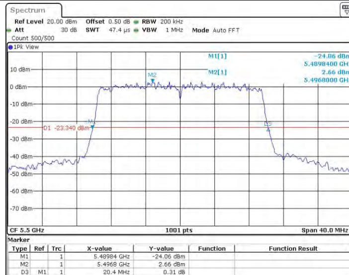
11AX20MIMO_Ant0_5500
