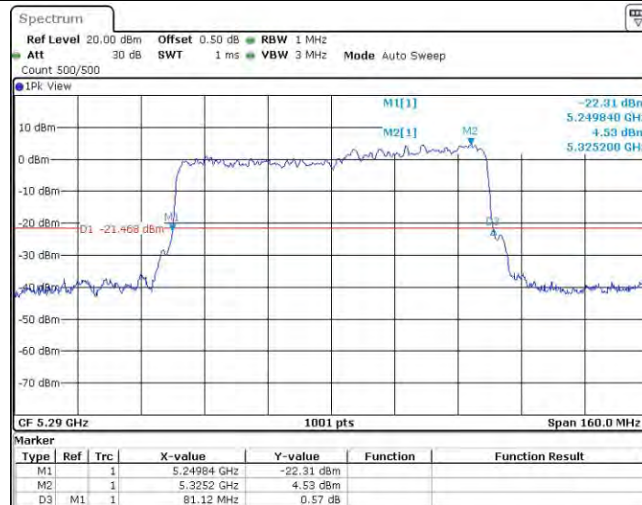
11AX80MIMO_Ant1_5290
