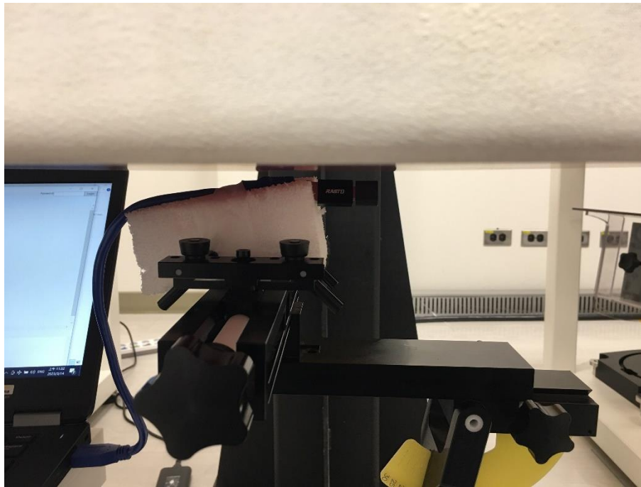
Vertical-Front
