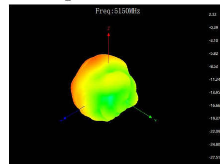
YZX face @5150MHz
