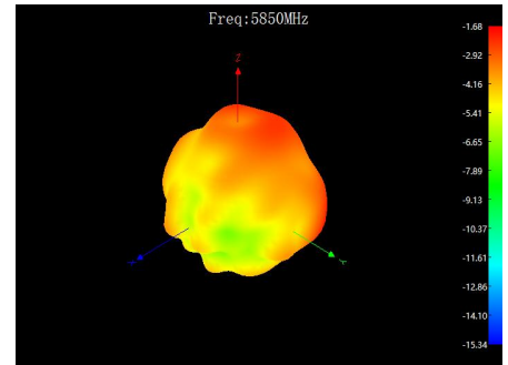
YZX face @5850MHz
