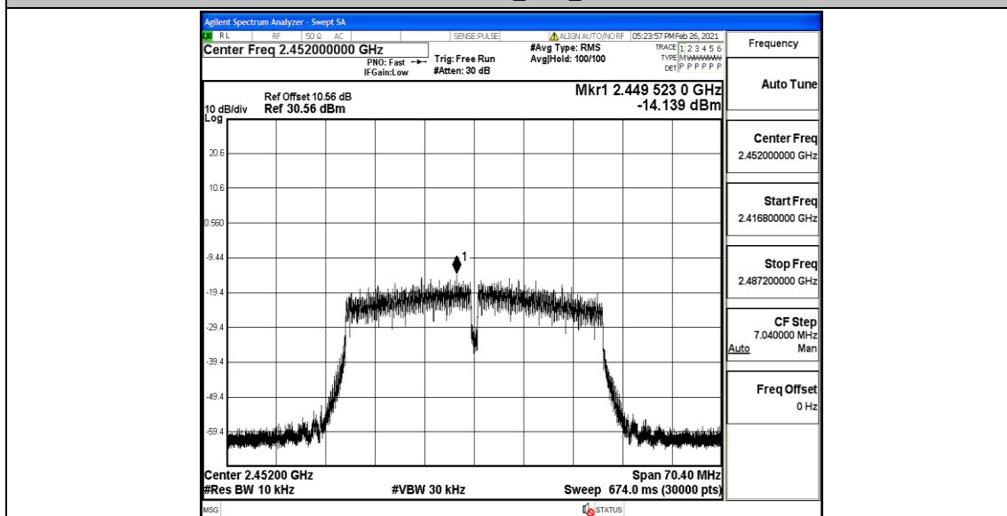
11N40MIMO_Ant2_2452
