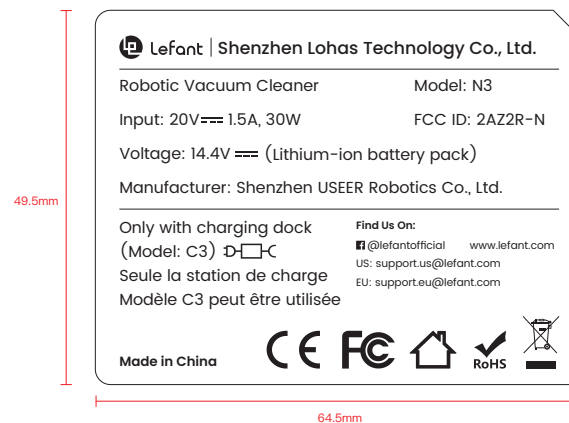
Lefant品牌 N3主机铭牌（欧美英通用）
