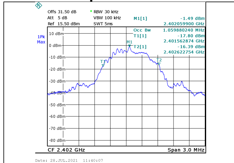
Figure 30. 2402.0 MHz, BLE
