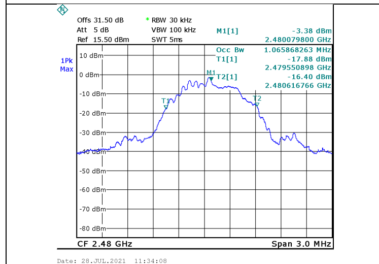
Figure 32. 2480.0 MHz, BLE
