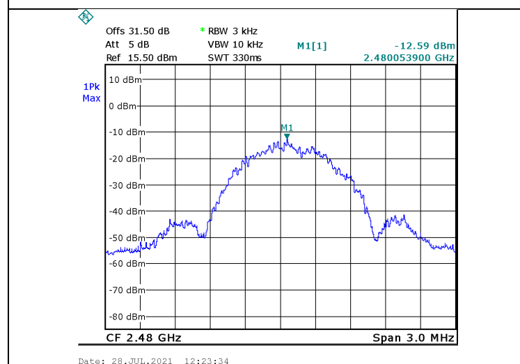
Figure 27. 2480.0 MHz, BLE
