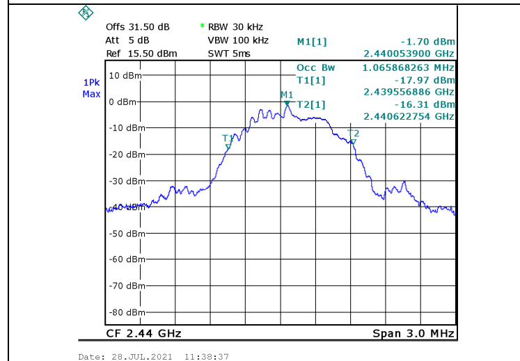
Figure 31. 2440.0 MHz, BLE
