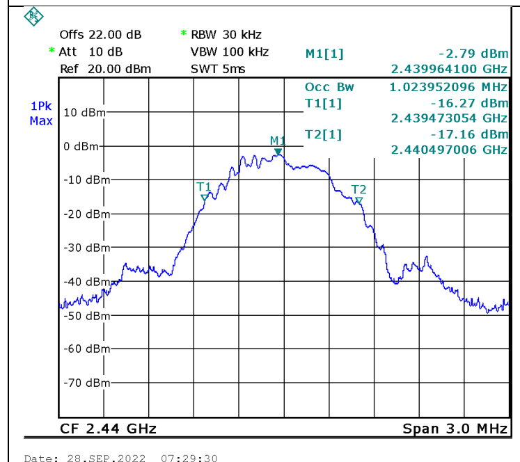
Figure 30. 2440.0 MHz, BLE
