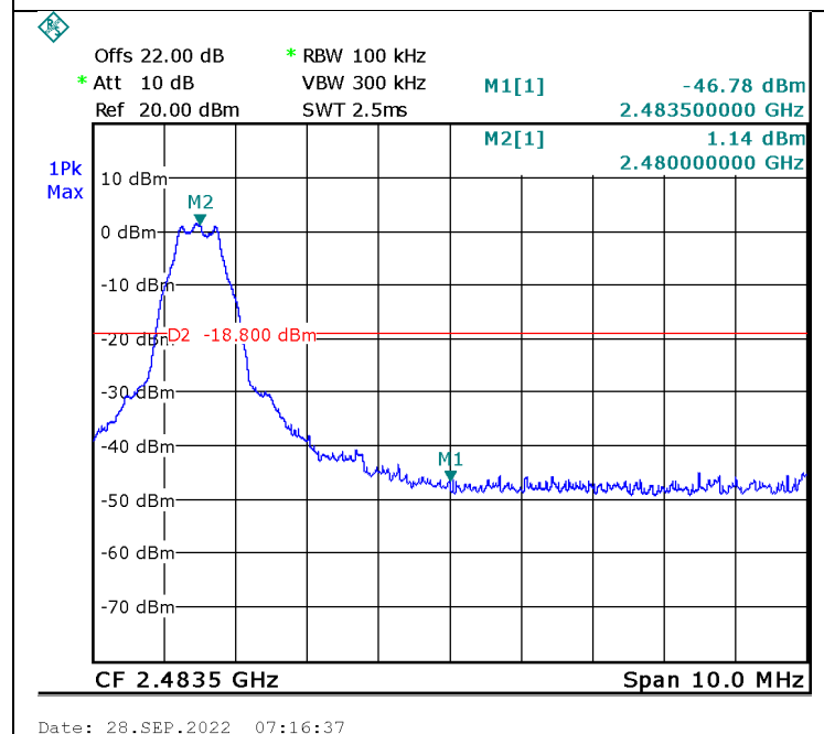
Figure 21. 2480.0 MHz, BLE
