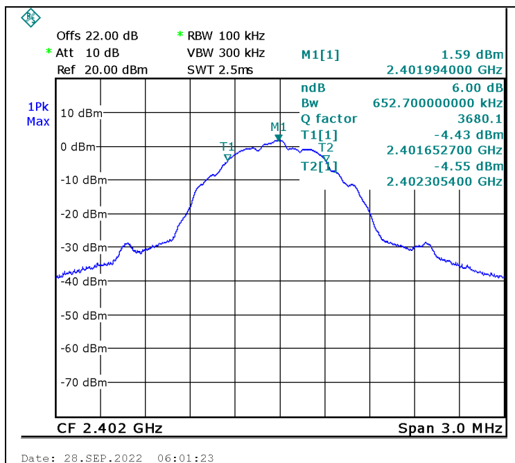
Figure 10. 2402.0 MHz, BLE
