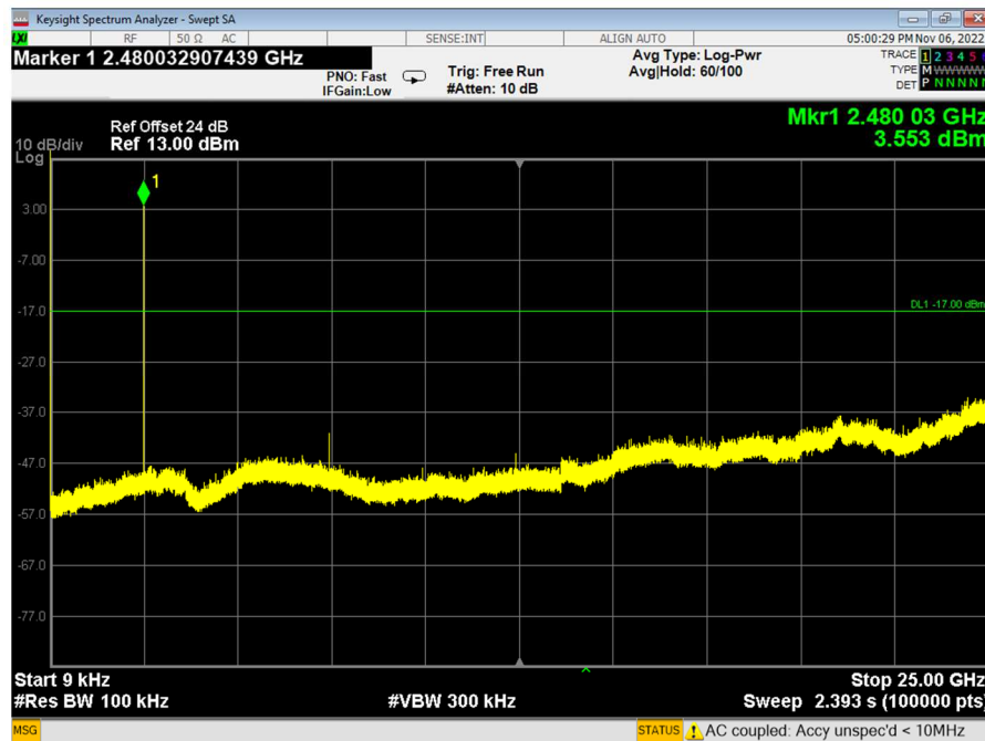
Figure 35 2480.0 MHz, BLE
