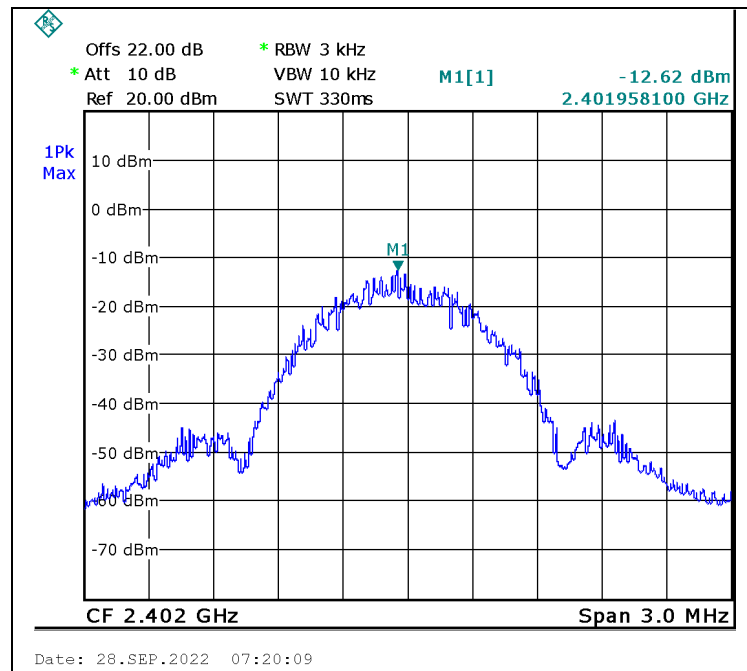
Figure 24. 2402.0 MHz, BLE
