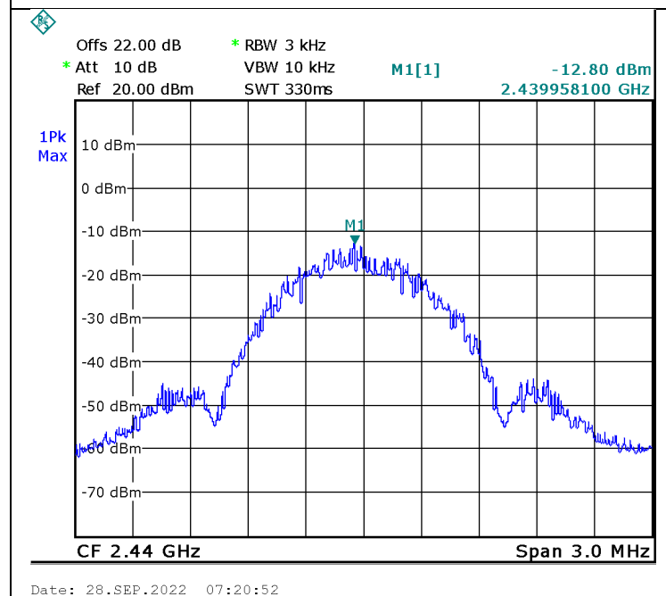
Figure 25. 2440.0 MHz, BLE
