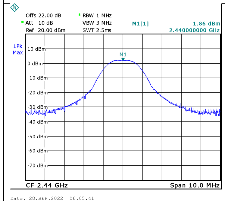
Figure 16. 2440.0 MHz, BLE
