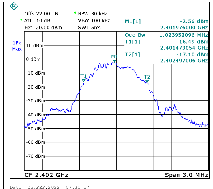
Figure 29. 2402.0 MHz, BLE
