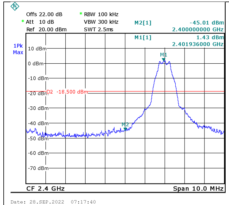
Figure 20. 2402.0 MHz, BLE
