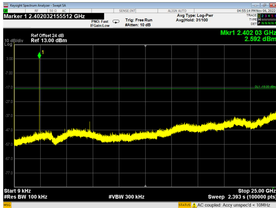
Figure 33 2402.0 MHz, BLE
