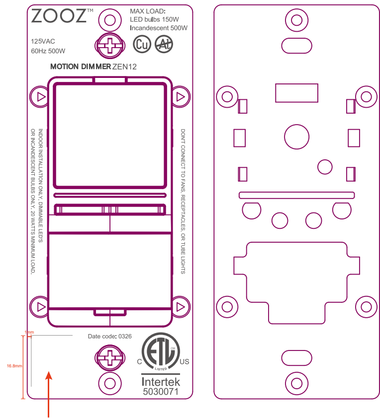
铝板图
